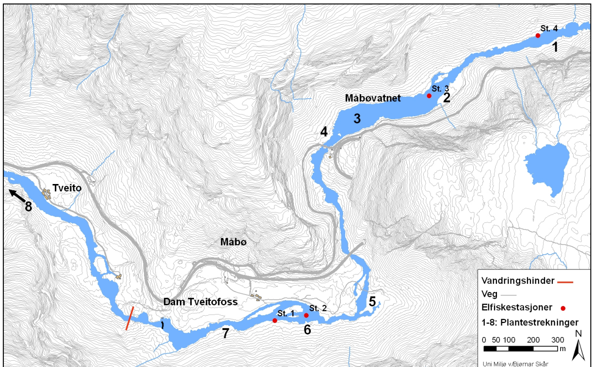
Figur 9. Oversikt over de viktigste lokalitetene for rognplanting (1-8) og stasjoner for elektrisk fiske (St. 1-4) på strekningen ovenfor Tveitofossen i Bjoreio.
