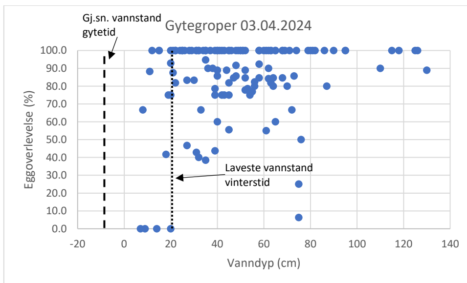
Figur 15. Sammenheng mellom vannndyp eggoverlevelse hos gytegroper undersøkt den 03.04.2024. Vannndypet angir dybden på gytegroppen ved tidspunktet de ble undersøkt. De to stiplede linjene viser henholdsvis viser den laveste vannstanden (døgnmiddel) registrert i løpet av inkubasjonstiden fra gyting og frem til undersøkelsene ble utført, og den gjennomsnittlige vannstanden i gytetiden om høsten i forkant (dvs. gytevannstand).
