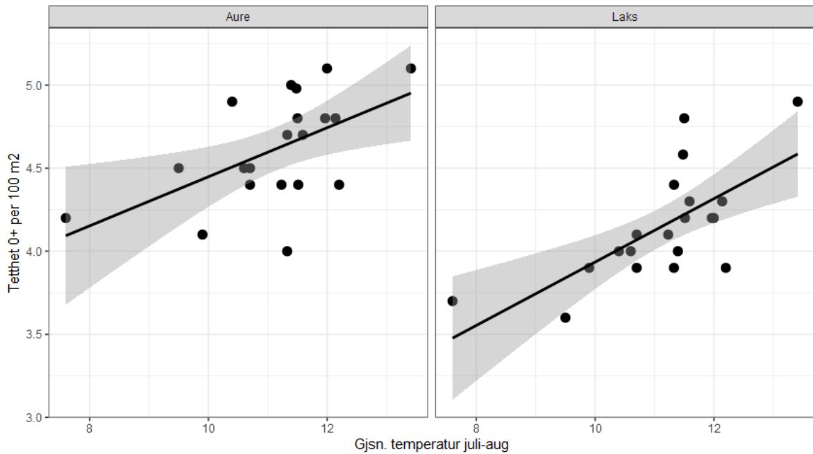
Figur 23. Sammenheng mellom vanntemperatur om sommer, gitt som gjennomsnitt i perioden juli-august, og fiskelengde hos ensomrig aure (t.v.) og laks (t.h.) i Bjoreio i perioden 2004-2023.
