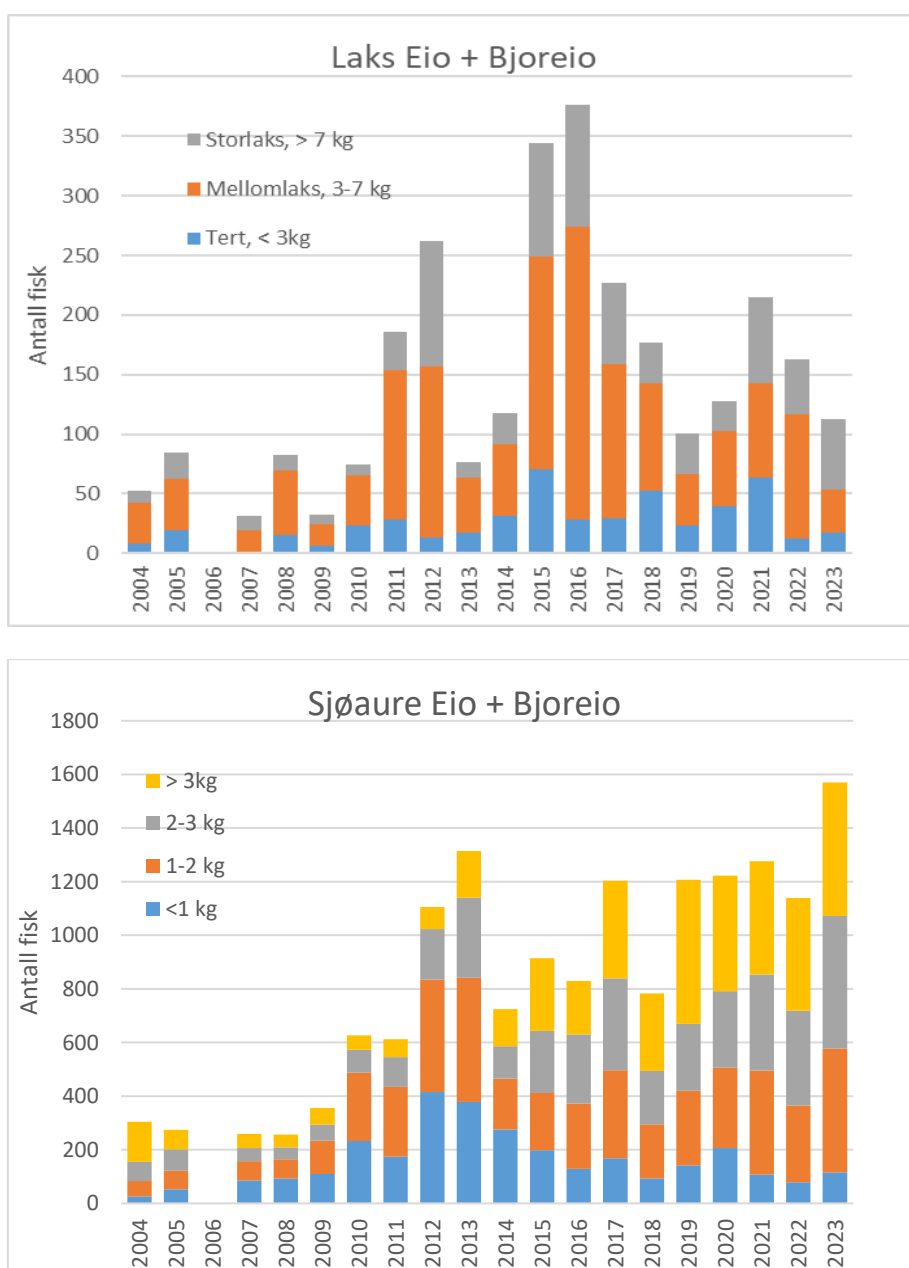
Figur 4. Antall laks (øverst) og sjøaure (nederst) av ulike størrelseskategorier registrert ved drivtelling av gytefisk samlet i Eio og Bjoreio i perioden 2004-2023. Data for Veig er utelatt siden det mangler data fra vassdragsavsnittet fra flere av årene i tidsserien.
