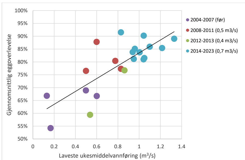
Figur 17. Sammenheng mellom den laveste ukesmiddelvanntføringen i løpet av vinteren (fra 1. november og frem til prøvetaking) og den gjennomsnittlige eggoverlevelsen registrert i gytegrøpene på våren. De ulike fargene indikerer hvilket manøvreringsreglement som har vært gjeldende i løpet av vintersesongen de ulike årene.
