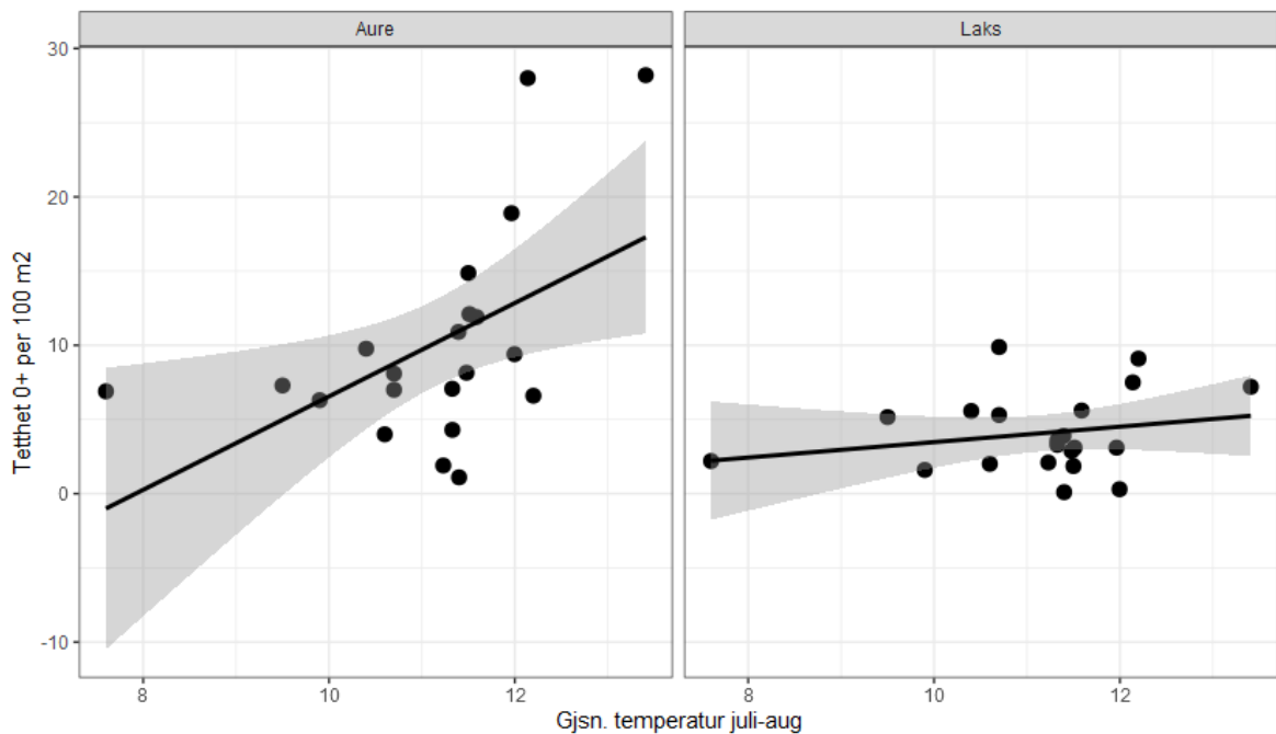
Figur 24. Sammenheng mellom vanntemperatur om sommer, gitt som gjennomsnitt i perioden juli-august, og tetthet av ensomrig aure og laks i Bjoreio i perioden 2003-2023. Linjen viser en lineær regresjonsmodell med 95 % konfidensintervall (grå skygge) for sammenhengen mellom temperatur og tetthet av fisk.
