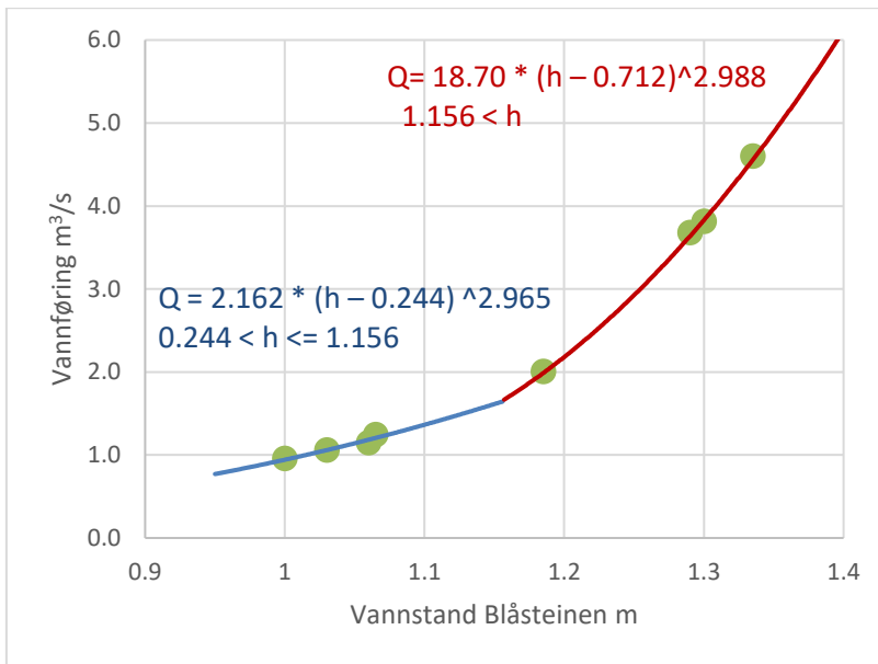
Figur 2. Sammenheng mellom vannstand og vannføring ved vannstandsloggeren ved Blåsteinen i Bjøreio. Sammenhengen er todelt og usikkerheten øker betydelig når vannstanden overstiger 1,4 m. De grønne punktene angir målinger av vannføring som sammenhengen er basert på, mens formlene angir beregning av vannføring for ulike vannstandsintervaller. Data oppgitt fra Statkraft.
