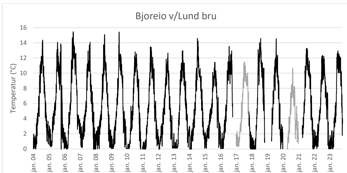
Figur 19. Døgnmiddel vanntemperatur i Bjoreio i perioden 2003-2022, med gjennomsnitt for perioden 2003-2021. Data er fra logger ved Lund bru bortsett fra 2017 og 2020 da data er basert på målinger ved Statkraft sin logger ved Blåsteinen (grå linje).
