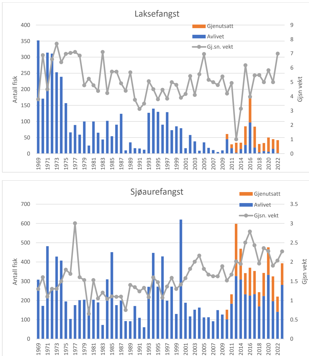
Figur 3. Fangststatistikk for laks (øverst) og sjøaure (nederst) i Eidfjordvassdraget i perioden 1969-2023. Laksen har vært fredet fra 2000 og utover, men det har vært tillatt å avlive oppdrettslaks. Gjenutsatt fisk har blitt rapportert siden 2010. Data fra lakseregistertet og www.fangstrapp.no .
