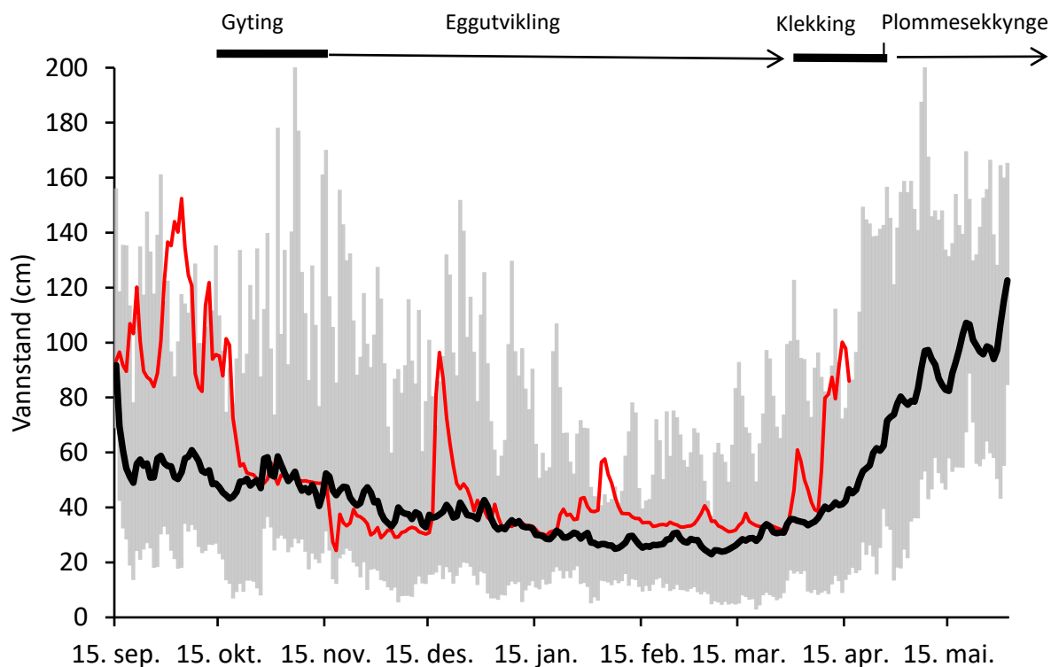
Figur 11. Vannstand (døgnmiddelnivå) i Bjoreio fra vannstandsloggerne ved Skarsenden i årene 2004-2011, og ved Blåsteinen i årene 2011-2024. Skalaen for vannstand (y-aksen) er standardisert slik at 0 cm tilsvarer en vannføring på 0 m 3 /s (dvs. stillestående vann på lokaliteten). Den svarte linjen indikerer gjennomsnittet i periodene, de grå søylene indikerer variasjonen i vannstands nivå i periodene. Den røde linjen viser vannstanden gjennom vinterhalvåret i 2023-2024, frem til 15. april 2024. Tidspunktet for gyting og inkubasjon er indikert øverst på figuren.
