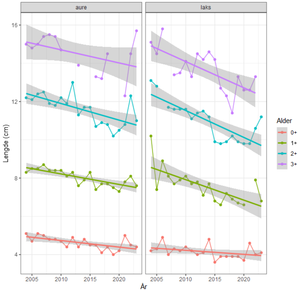
Figur 25. Gjennomsnittlig lengde på ungfisk av ulike aldersgrupper av laks (t.h.) og sjøaure (t.v.) fra ungfiskundersøkelser i Bjoreio i perioden 2004-2023. Linjene viser synkende trend over tid analysert for hver enkelt årsklasse (lineære regresjonsanalyser, alle p < 0,05 ).
