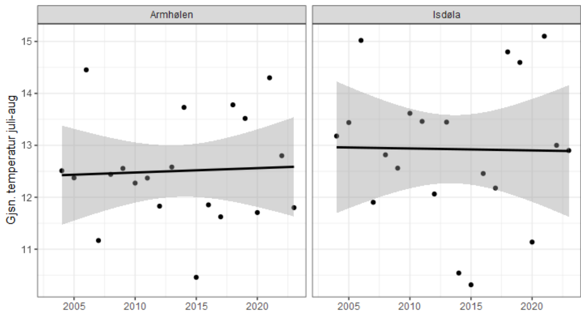
Figur 26. Gjennomsnittlig vanntemperatur i sommerperioden juli-august på anadrom strekning i Bjoreio i perioden 2004-2023. Linjen viser trenden over tid fra en lineær regresjonsmodell med 95 % konfidensintervall. Pilen indikerer perioden det er vært drift i Leiro kraftverk (fra 2011).
