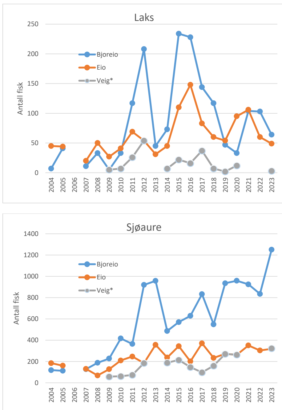
Figur 5. Oversikt over antall laks (øverst) og sjøaure (nederst) observert ved drivtelling i de ulike vassdragsavsnittene i Eidfjordvassdraget i undersøkelsesperioden. *I Veig foreligger kun data for deler av perioden.
