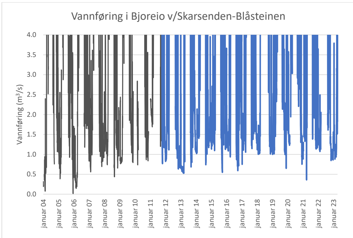
Figur 12. Vannføring på døgnmiddelnivå i Bjoreio ved Skarsenden i perioden 2004-2011 (svart kurve) og ved Blåsteinen i perioden 2011-2024 (blå kurve). Kurvene for lokalitetene er kun etablert for lave vannføringer, og viser vannføringer < 4 m 3 /s.
