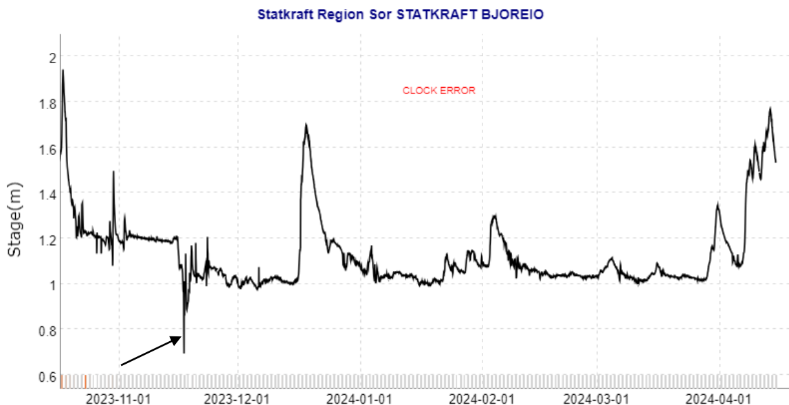
Figur 14. Vannstand i Bjoreio på timesbasis fra vannstandsloggeren ved Blåsteinen vinteren 2023/2024. Pilen viser en irregulærhet i vannstand forårsaket av driftsendring i Tveitafossen kraftverk.
