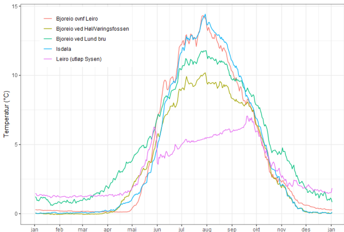
Figur 20. Vanntemperatur (døgnmiddel) for i perioden 2001-2023 med tilgjengelige data fra Bjoreio ovenfor Leiro (Armhølen), Leiro like nedstrøms tappeventilen i Sysendammen, Isdøla, Bjoreio ved Høl (Vøringsfossen) og Bjoreio på lakseførende strekning ved Lund Bru.
