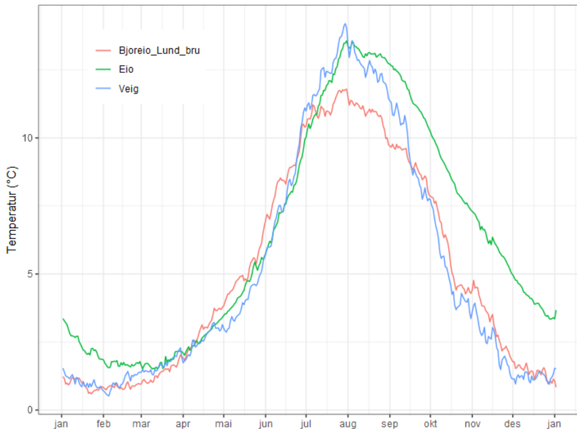
Figur 18. Flerårsgjennomsnitt av døgnmiddel vanntemperatur i Veig, Bjoreio og Eio i perioden 2009-2023.
