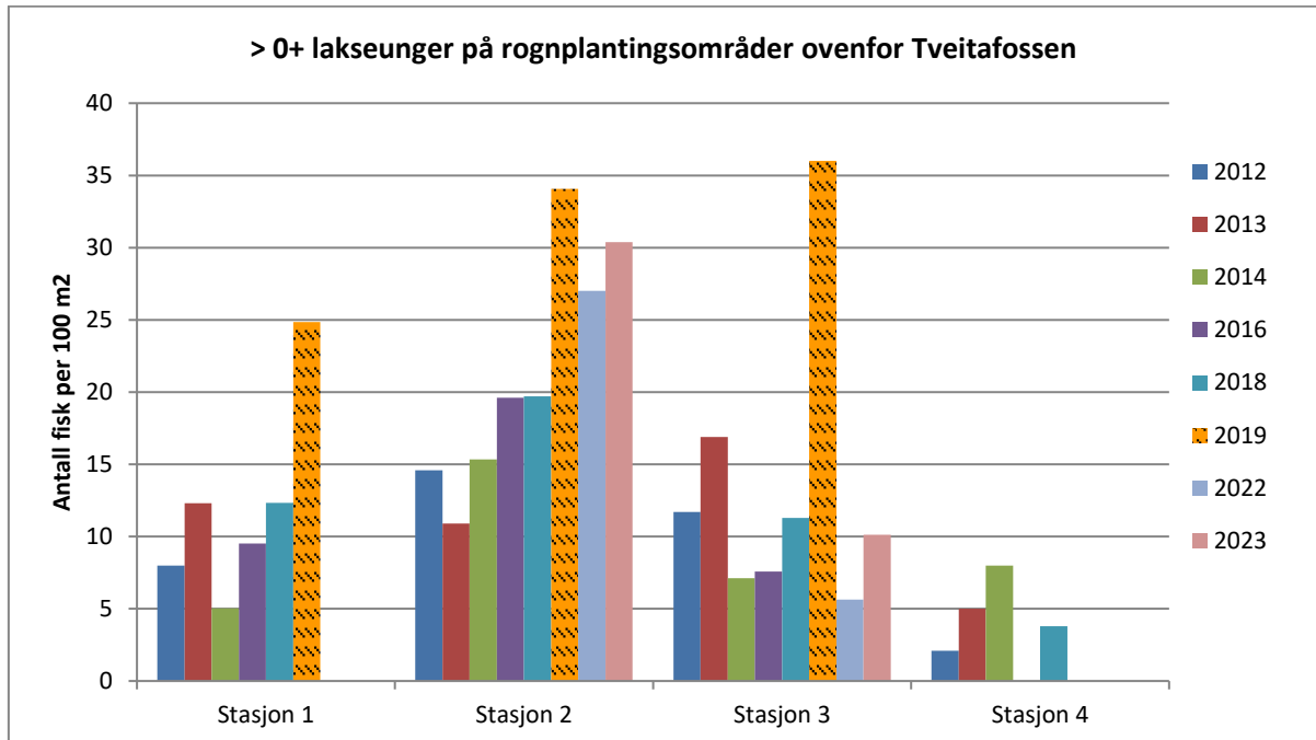
Figur 10. Tettheter av eldre (>0+) lakseunger på de fire stasjonene på rognplantingsområdene oppstrøms Tveitafossen i Bjoreio. Data fra Statkraft.
