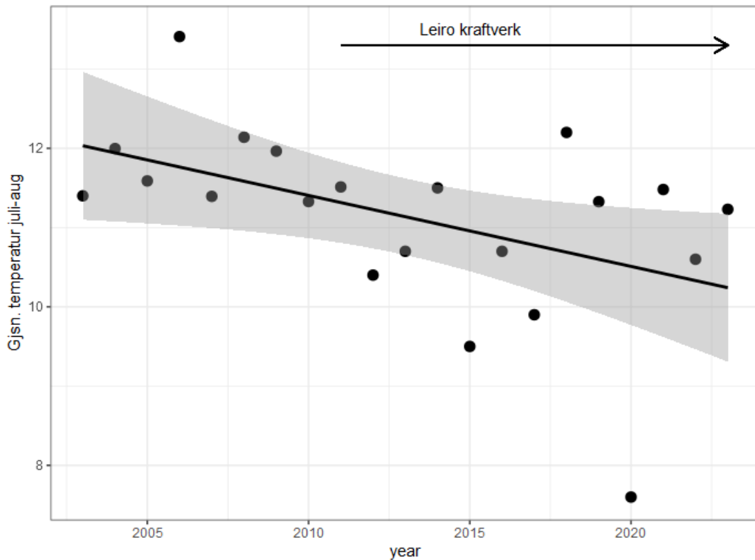
Sommertemperatur i Bjoreio v/Lund bru
