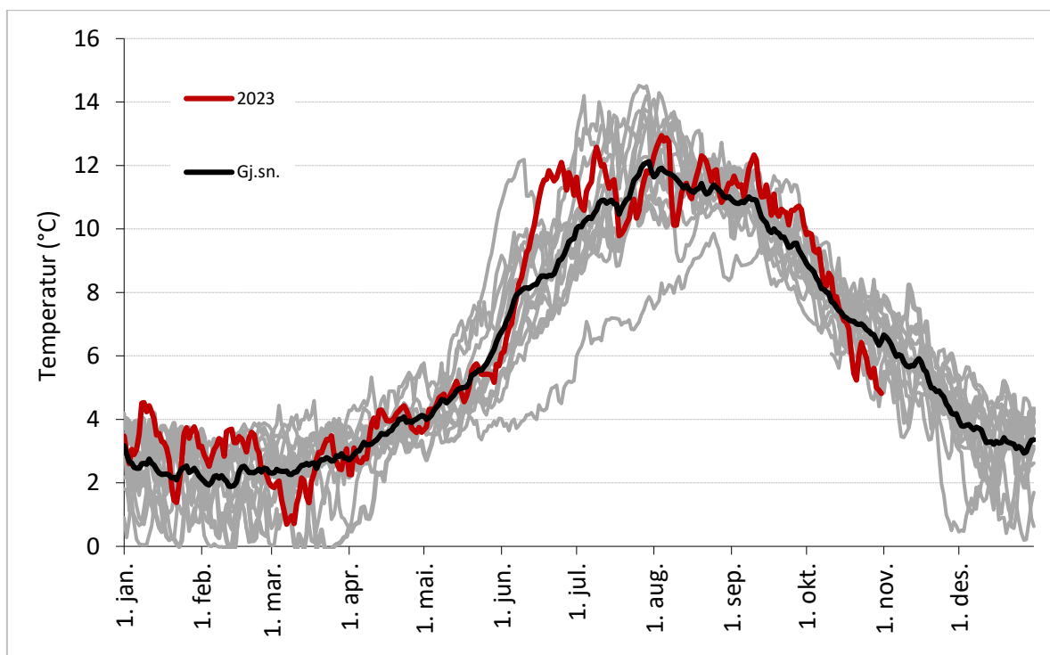
Figur 21. Døgnmiddel vanntemperatur i Øyreselva i perioden 2008-2023. Data for 2023 er markert i rødt, mens grå linjer er data for de enkelte år tidligere i perioden.
