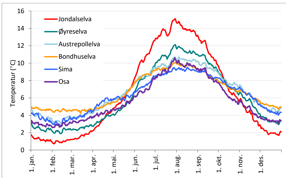
Figur 4. Gjennomsnittlig vanntemperatur på døggnivå fra de seks regulerte elvene i Hardanger i perioden 2007-2023.
