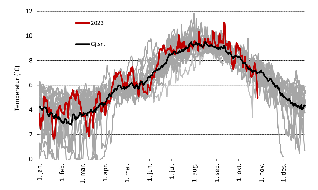
Figur 6. Døgnmiddeltemperaturer fra loggere i Sima i perioden 2008-2023. Data for 2023 er markert i rødt, mens grå linjer er data for de enkelte år tidligere i perioden. Temperaturer under 0 grader tyder på at loggeren ved enkelte anledninger har vært tørrlagt i kortere perioder på vinteren i noen år.
