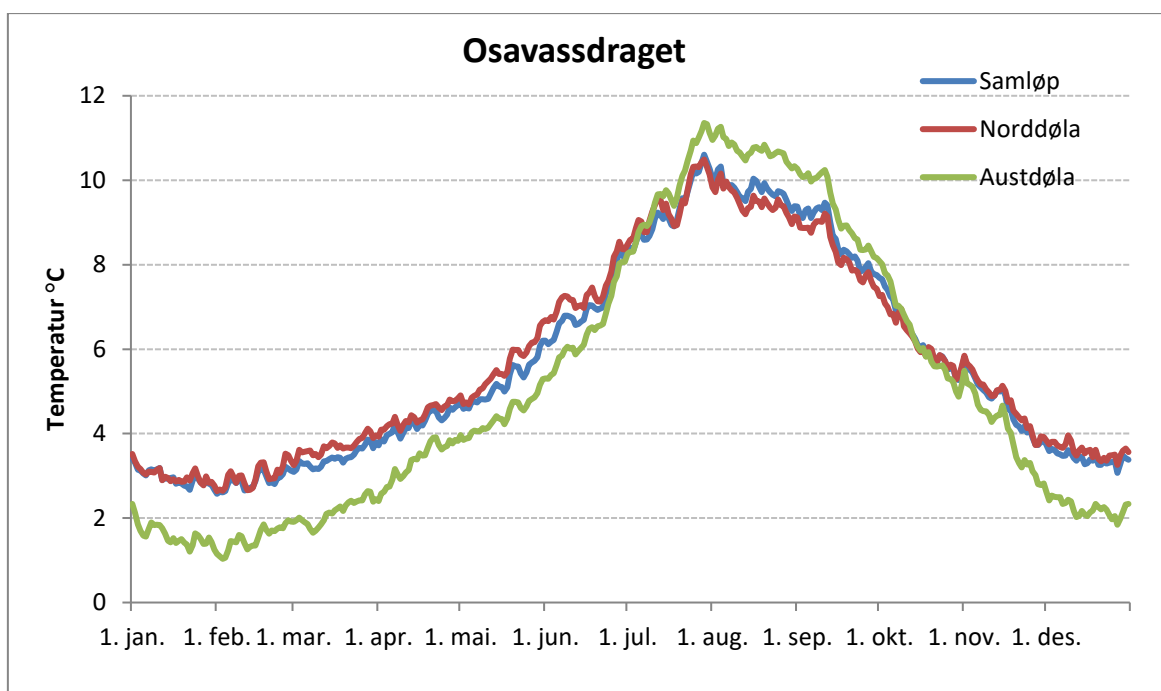
Figur 10. Døgnmiddeltemperaturer (gjennomsnitt for døgn) i de ulike vassdragsavsnittene i Osavassdraget i perioden 2008-2023.
