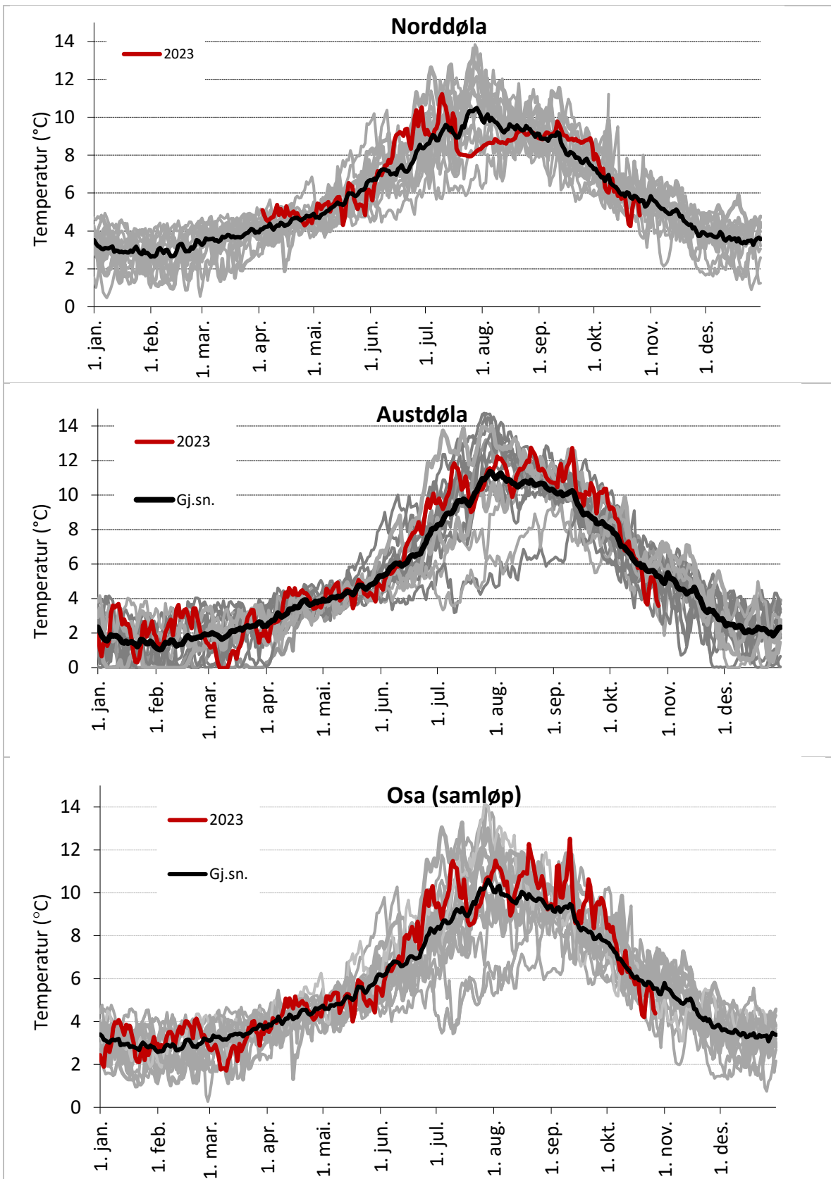
Figur 11. Døgnmiddeltemperatur i Norddøla (øverst), Austdøla (midten) og samløpet (nederst) i 2008-2023. Data for 2023 markert i rødt, mens grå linjer er data for de enkelte år tidligere i perioden.
