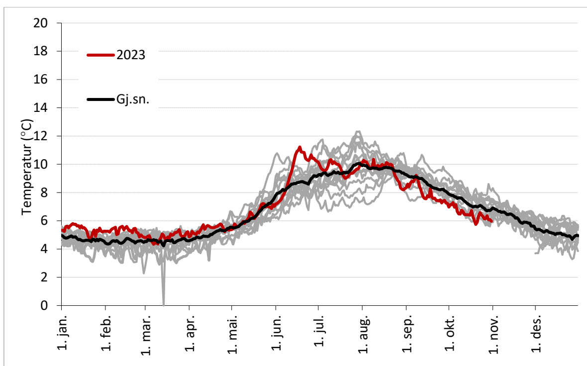
Figur 29. Døgnmiddeltemperatur i Bondhuselva i perioden 2008-2023. Data fra 2023 er markert i rødt, mens de grå linjene indikerer data fra enkeltår tidligere i perioden.
