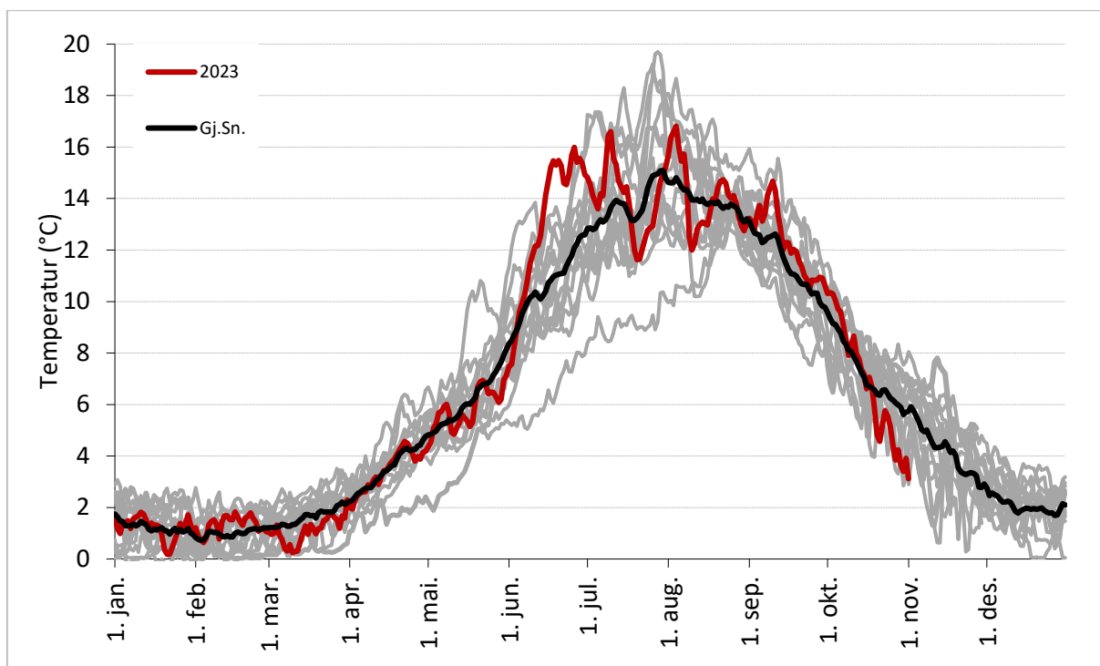
Figur 16. Døgnmiddeltemperatur i Jondalselva i perioden 2008-2023. Data for 2023 er markert i rødt, mens grå linjer er data for de enkelte år tidligere i perioden.
