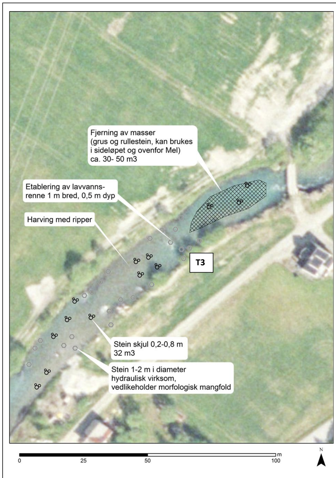
Figur 23. Arbeidsbeskrivelse med prinsipiell utforming i plan for tiltaksområde 2.1 Nedrebø.
