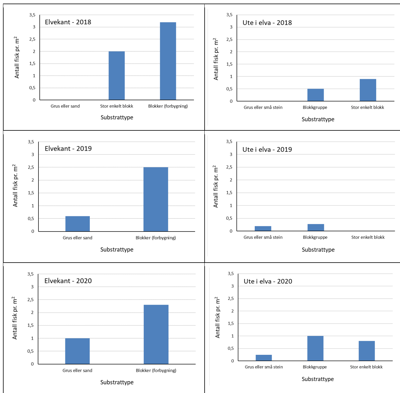
Figur 25. Tettheter av ungfisk basert på et punktfiske med elektrisk fiskeapparat i ulike typer substrat i elvekant (øverst) eller ute i elva (nederst) i perioden 2018- 2020.
