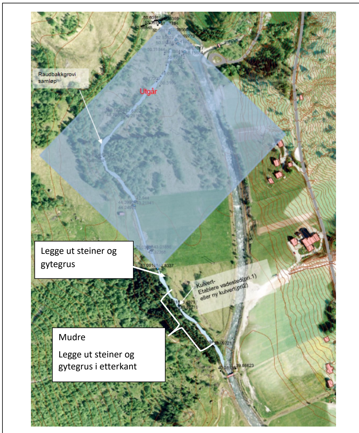
Figur 15. Revidert plantegning av forslag til habitattiltak i nedre del av Raudbakkgrovi. Alle punkter er oppmålte høydedata (moh.).
