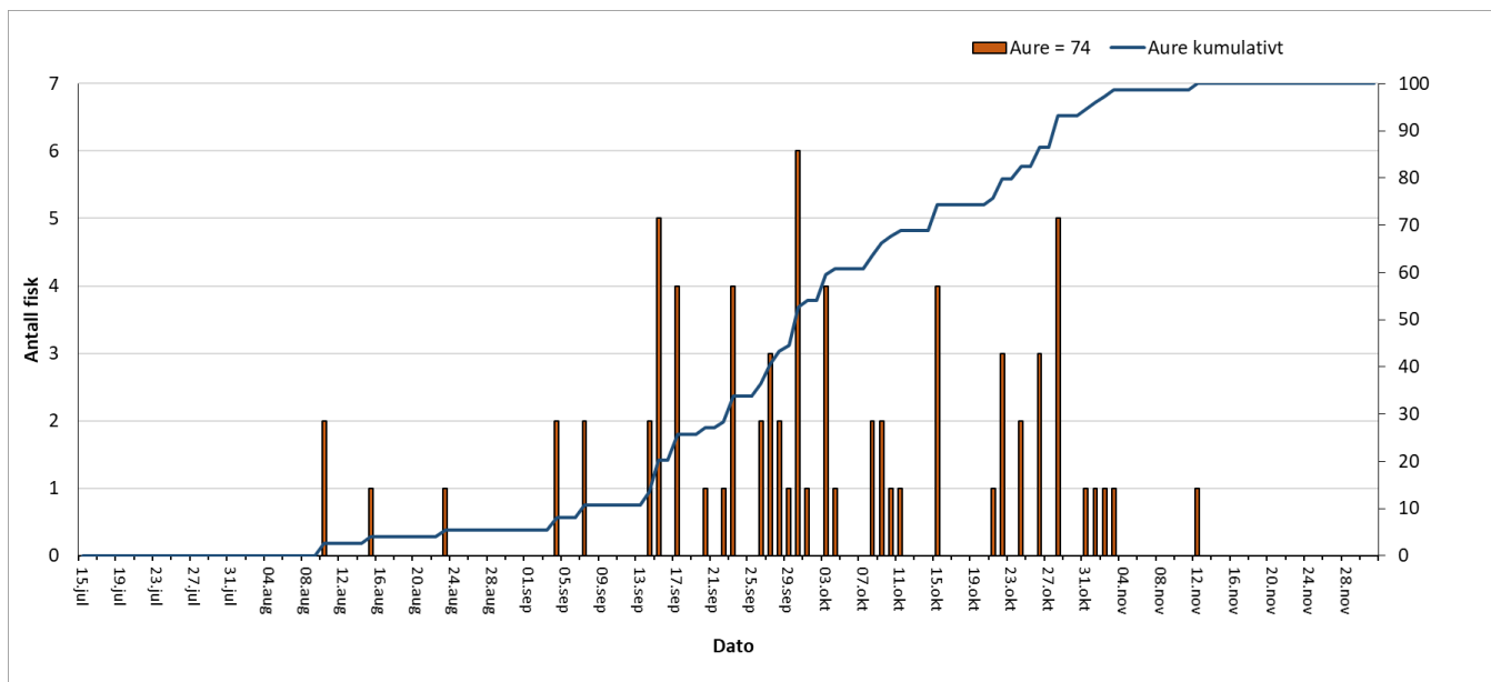
Figur 28. Overvåking av gytefisk av sjøaure som vandret opp fisketrappen i Vetlefjorden i perioden 15.07.2020 til 01.12.2020.
