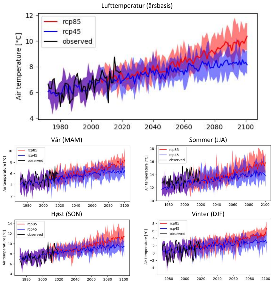
Figur 6.1. Modellert lufttemperatur 1970-2100 projisert på Håelvas nedbørfelt, basert på 10 kombinasjoner av globale og regionale klimamodeller og to scenarioer for utslipp av klimagasser (RCP4.5 og RCP8.5). De tykke røde og blå linjene representerer gjennomsnittet for de 10 modellkombinasjonene, mens det skraverte arealet viser variasjonen mellom de individuelle modellene. Øverste panel viser årlige gjennomsnitt, mens de nederste panelene viser resultatene fordelt på sesonger.
