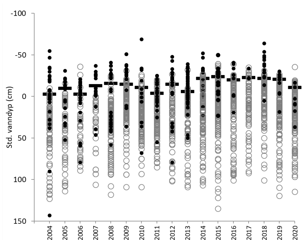
Figur 18. Eggoverlevelse i undersøkte gytegrøper i forhold til vanndyp og laveste vannstand i Bjoreio i perioden 2004-2020. Åpne sirkler angir gytegrøper med normalt høy overlevelse (>50 %), mens svarte sirkler angir gytegrøper med lav eggoverlevelse (< 50 %). Vannføringen er standardisert slik at det viser samme nivå for de ulike årene, og der en vannstand lik 0 tilsvarer en vannføring nær 0. De svarte linjene indikerer den laveste vannstanden (på døgnnivå) som forekom i løpet av vinteren i de ulike årene, dvs. gytegrøper som ligger på oversiden av linjen har sannsynligvis vært utsatt for tørrlegging.
