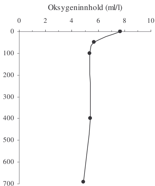
Figur 3.1. Temperatur, saltholdighet og oksygen. Temperatur og saltholdighet er målt med CTD-sonde fra overflaten og til 700 meter dyp mens og oksygeninnhold (ml/l) er målt med Winkler-metode i vannprøver fra seks dyp fra overflaten og til 700 meter på stasjon Vind 4 den 21. februar 2008.
