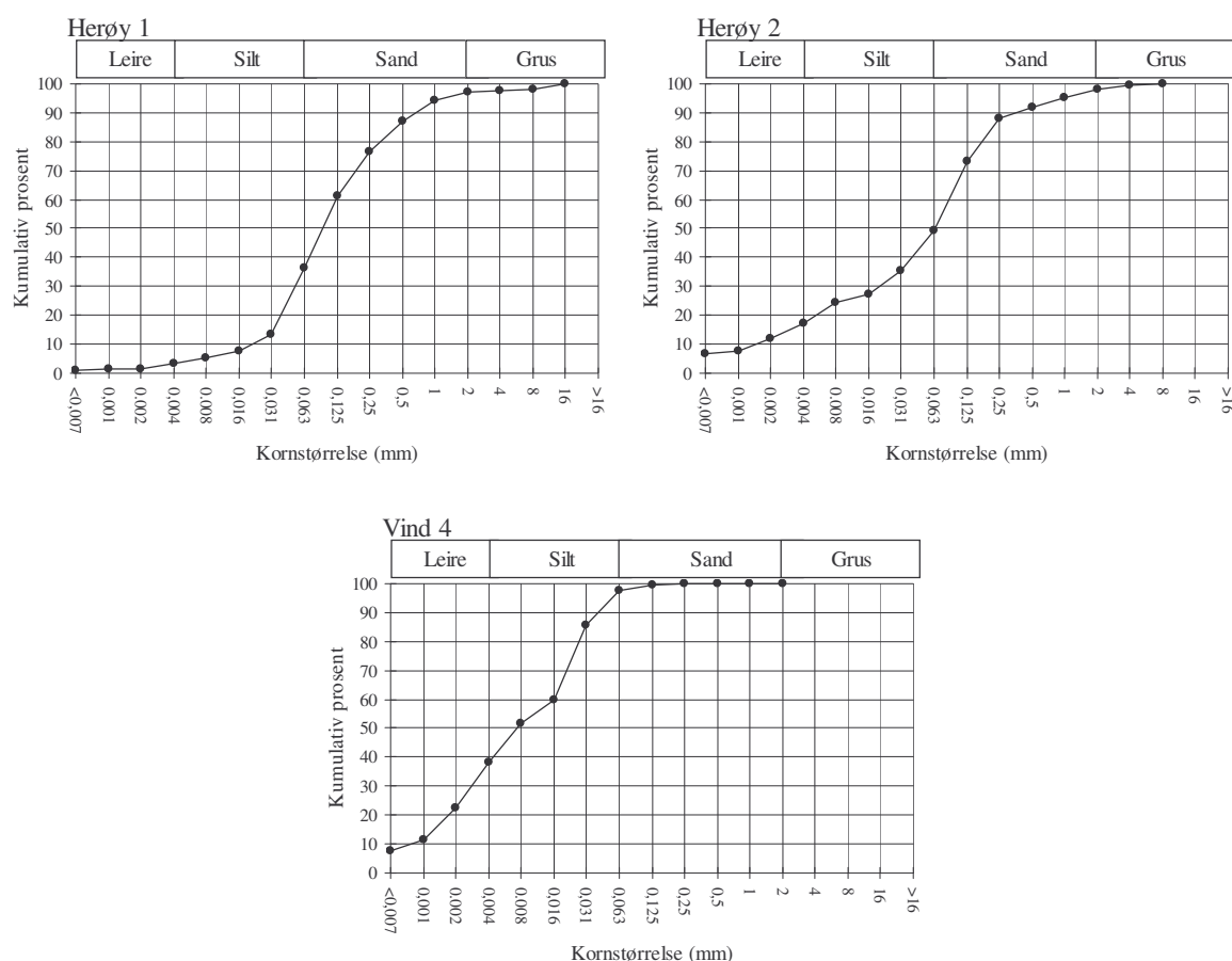
Figur 3.2. Kornfordeling (mm) langs x-aksen og kumulativ vektprosent langs y-aksen av sedimentprøver fra Herøy og Vindafjorden i 2008.
