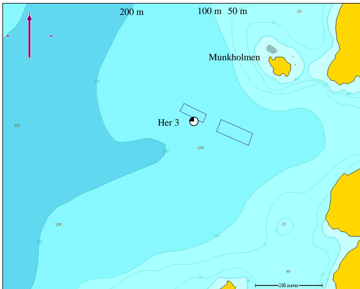
Figur 2.3. Detaljskisse over lokaliteten med stasjonen i nærsonen og en enkel skisse av anlegget. Eksakt plassering av stasjonen er gitt i Tabell 2.1. Vurdering av miljøforholdene på stasjonen er markert med kakediagram, der ○ = svært bra, ◐ = bra, ◑ = middels, ◒ = dårlige miljøforhold og ◓ = dødt. Kartkilde: Olex.
