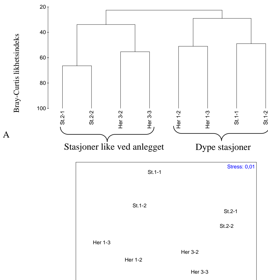
Figur 3.4. De multivariate analysene viste at det var stor likhet mellom de to huggene fra hver enkelt stasjon, men stor forskjell i faunasammensetningen mellom stasjonene. A) Cluster og B) MDS-plot med stressfaktor 0,01. Beregningene er foretatt på fjerderots-transformerte artsdata. Bassert på Bray-Curtis indeks. Stasjonene merket med St er fra innsamlinga i januar 2007, mens stasjonene merket med Her er fra innsamlinga i desember 2007. Her 1-1: 1. hugg fra stasjon Her 1.
