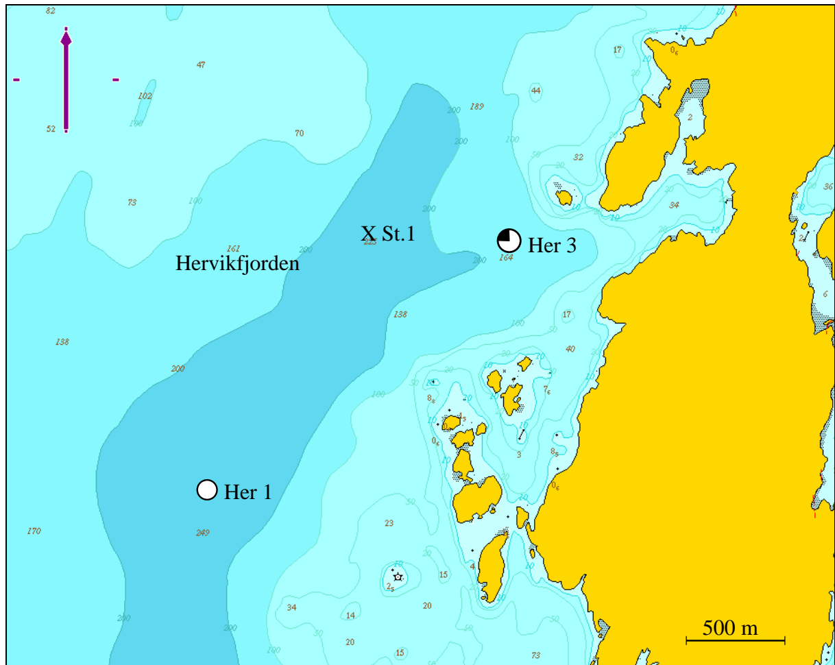
Figur 2.2. Utsnitt av Hervikfjorden med referansestasjonen i dypet og stasjonen ved anlegget. Eksakt plassering av stasjonene er gitt i Tabell 2.1. Vurdering av miljøforholdene på stasjonene er markert med kakediagram, der ○ = svært bra, ◐ = bra, ◑ = middels, ◒ = dårlige miljøforhold og ◓ = dødt. Kartkilde: Olex. St. 1: Stasjon fra innsamlingen til Bio Consult i januar 2007.
