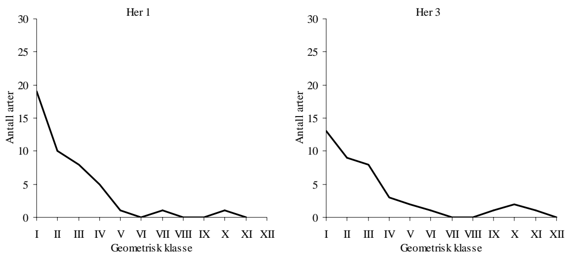
Figur 3.3. Antall arter langs (y-akse) er plottet mot geometriske klasser (x-akse) i prøvene fra Munkholmen.
