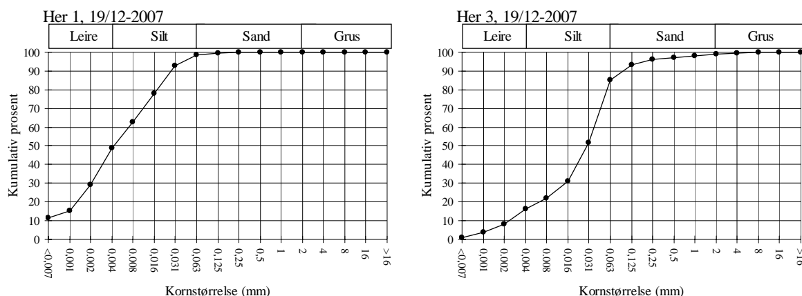
Figur 3.2. Kornfordeling (mm) langs x-aksen og kumulativ vektprosent langs y-aksen av sedimentprøver fra Munkholmen i 2007.
