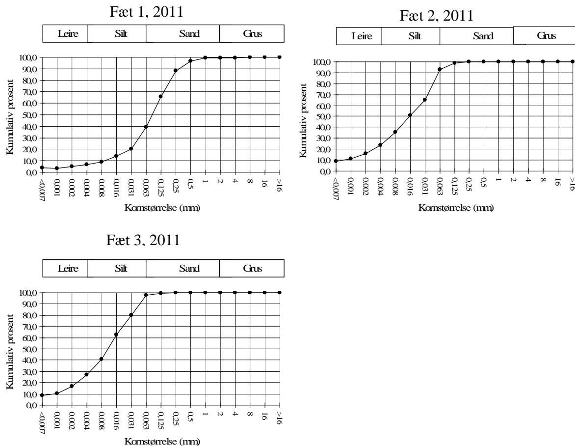
Figur 3.1. Kornfordeling (mm) langs x-aksen og kumulativ vektprosent langs y-aksen av sedimentprøver fra stasjonene Fæt 1, Fæt 2 og Fæt 3.
