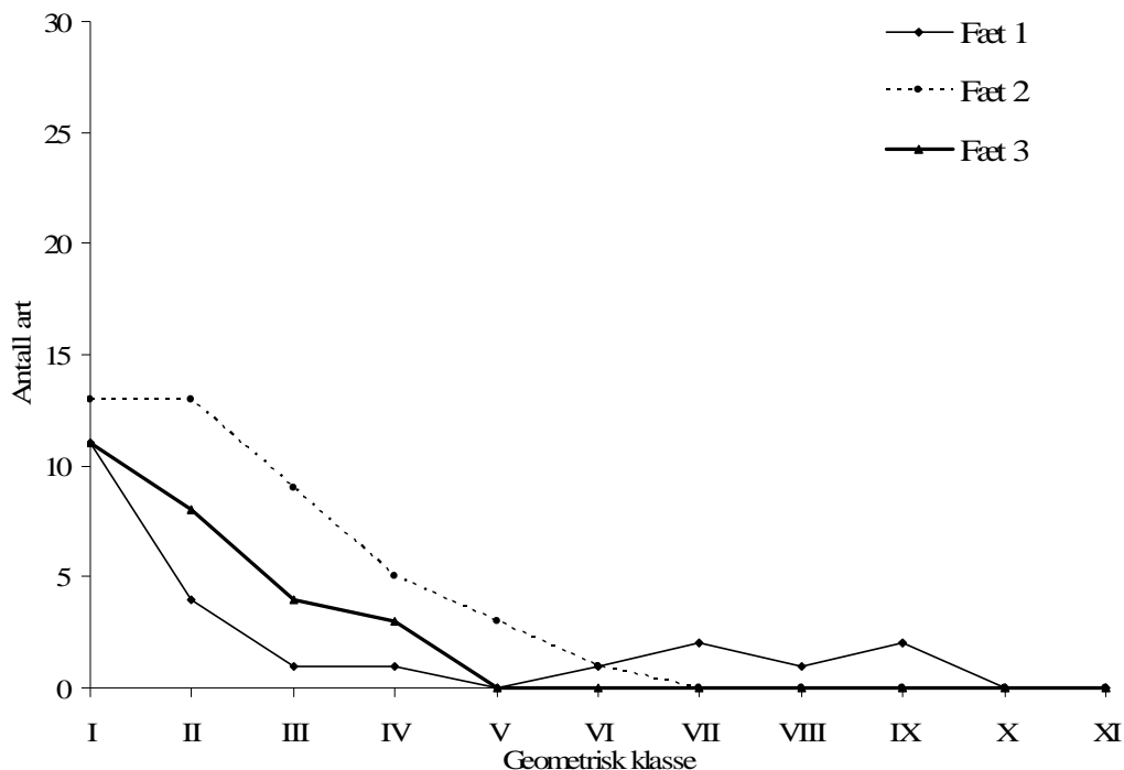
Figur 3.2. Antall arter langs (y-akse) er plottet mot geometriske klasser (x-akse) i prøvene.
