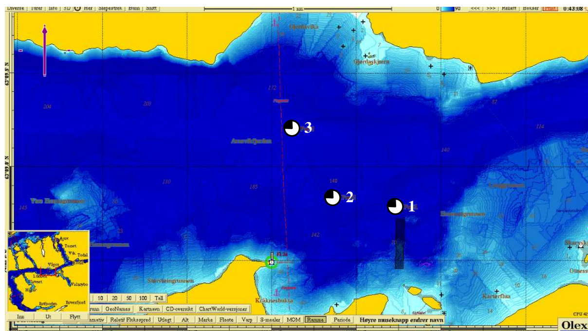
Figur 2.1. Oversiktskart med fjordsystemet på Nord-Møre (innfelt) og mer detaljert over området rundt Fætten, Vinjefjorden (hovedbilde). Vurdering av miljøforholdene er vist kom kakediagram, der ○ = svært bra, ◐ = bra, ◑ = middels, ◒ = dårlige miljøforhold og ◓ = dødt. Kartkilde: Olex
