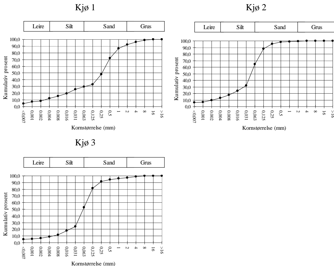
Figur 3.1. Kornfordeling (mm) langs x-aksen og kumulativ vektprosent langs y-aksen av sedimentprøver fra stasjonene ved Kjørsvikgrunnen i 2011.
