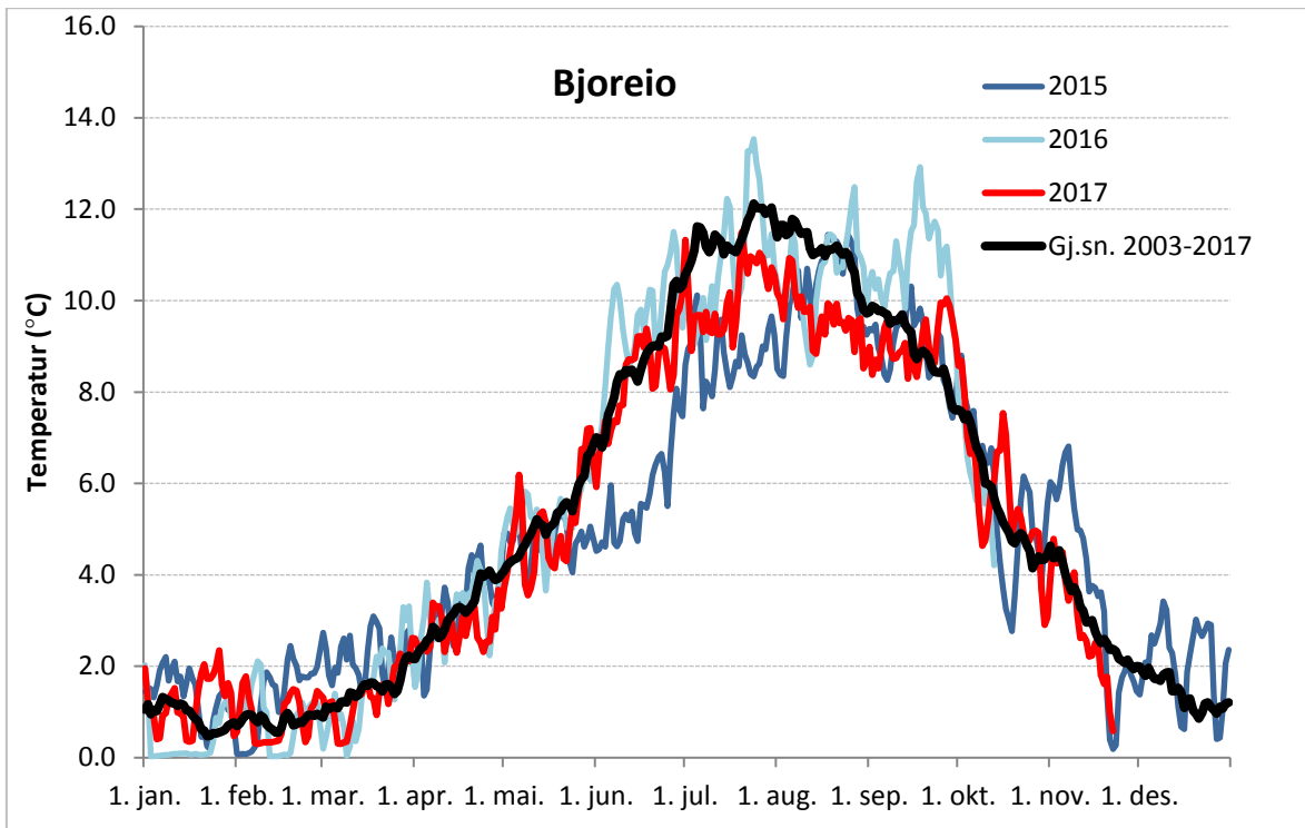
Figur 21. Døgnmiddel vanntemperatur i Bjoreio i perioden 2014-2017, med gjennomsnitt for perioden 2003-2017. I perioden 2003-2016 er målingene gjort ved Lund bru. Siden loggeren forsvant i 2017 er dataene fra dette året hentet fra vannstandsstasjonen ved Blåsteinen.
