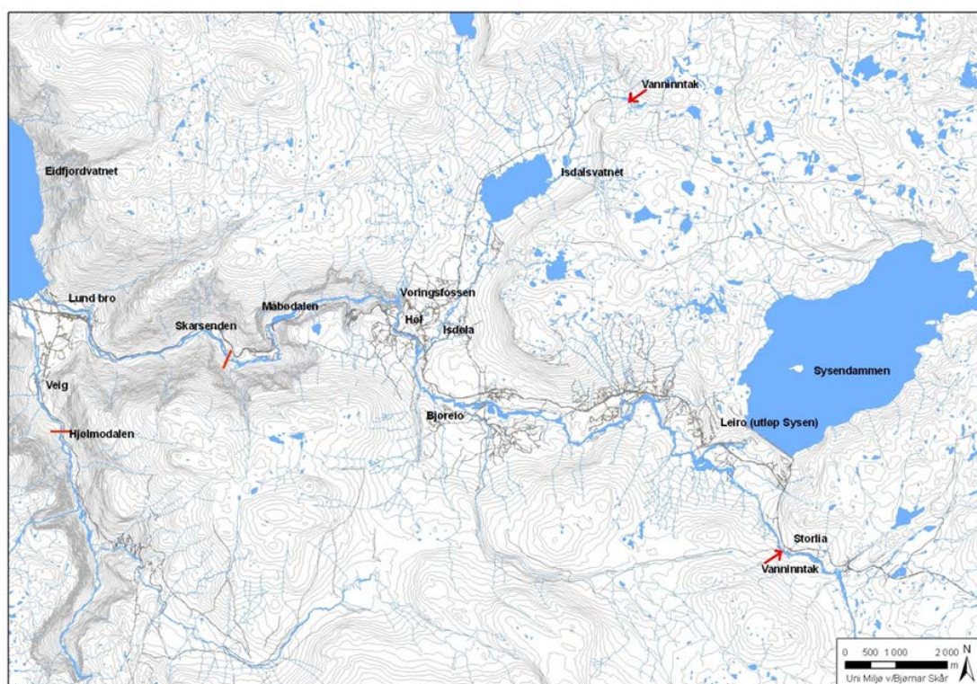
Figur 25. Kart over tilsigsområdet til Bjoreio. Lukene hvor vann fra Isdal og Storlia slippes fra er markert med piler.
