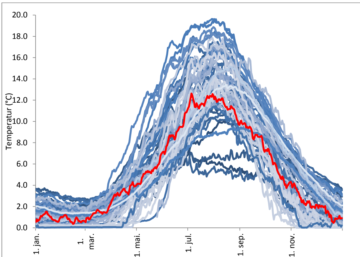
Figur 22. Gjennomsnittlig temperatur (døgnnivå) i Bjoreio sammenliknet med 63 andre lakseførende vassdrag i Norge. Bjoreio er indikert med rød linje.
