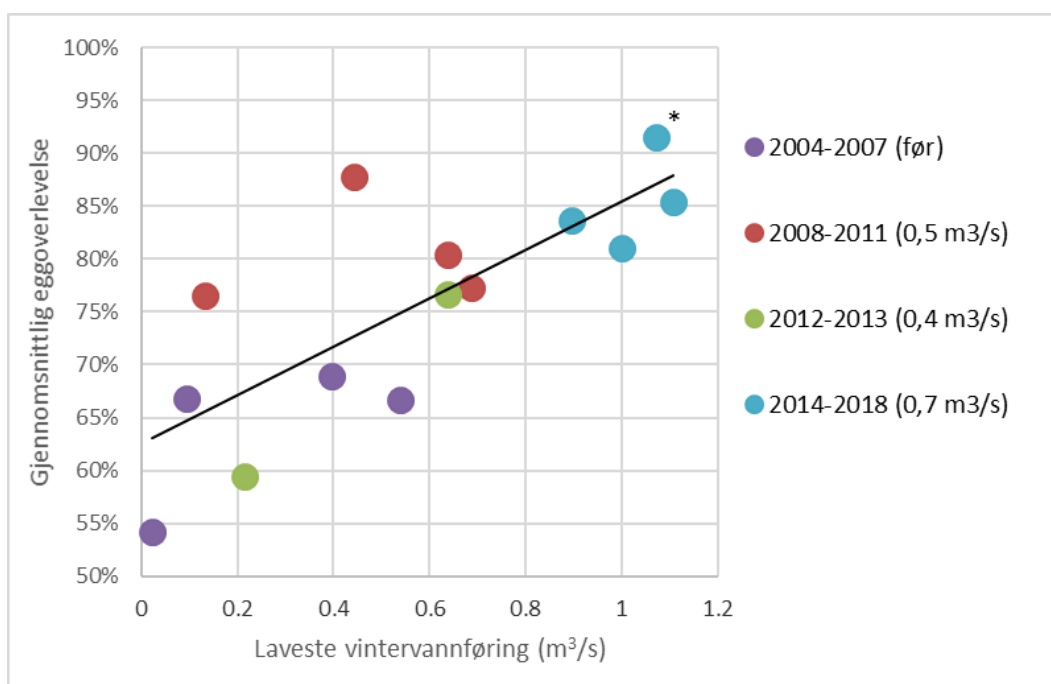
Figur 18. Sammenheng mellom den laveste vannføringen som forekommer i løpet av vinteren frem til prøvetaking og den gjennomsnittlige eggoverlevelsen registrert i gytegroperne på våren. De ulike fargene indikerer hvilket manøvreringsreglement som har vært gjeldende i løpet av vintersesongen de ulike årene. *Lavere vannføringsverdier som forekom under gytetiden i 2016, samt som følge av islegging og/eller stans i Tveitafoss kraftverk vinteren 2017, er utelatt.
