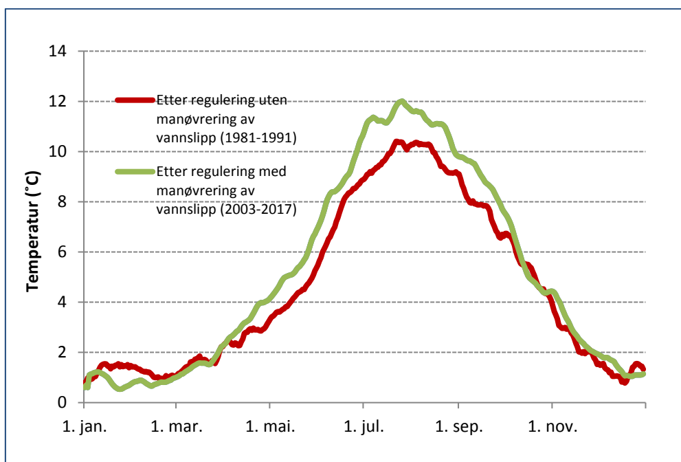
Figur 27. Gjennomsnittlig vanntemperatur på lakseførende strekning i Bjoreio (løpende gjennomsnitt for uke) for perioden etter regulering før manøvrering av vannslipp fra Storlia (1981-1991), og etter at vannslippet har blitt gjennomført.
