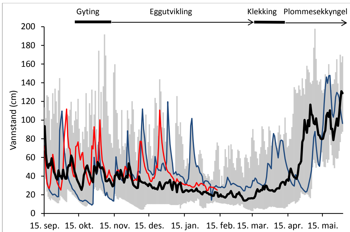
Figur 13. Vannstand (døgnmiddelnivå) i Bjoreio fra vannstandsloggerne ved Skarsenden (2004-2011) og Blåsteinen (2011-2017). Skalaen for vannstanden er standardisert slik at 0 cm tilsvarer en vannføring på 0 m 3 /s (dvs. stillestående vann på lokaliteten). Den svarte linjen indikerer gjennomsnittet i perioden, de grå søylene indikerer verdiene for høyeste og laveste vannstands nivå i perioden. Den blå og røde linjen viser vannstanden gjennom vinterhalvåret i henholdvis 2016-2017 og så langt i 2017-2018. Tidspunktet for gyting og inkubasjon er indikert øverst på figuren.
