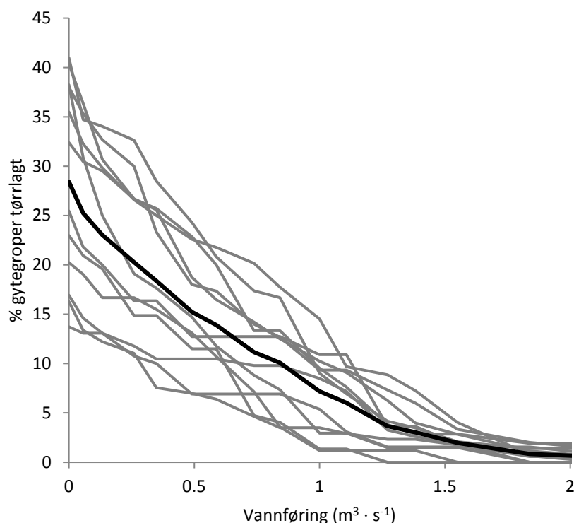
Figur 19. Forventet andel av gytegroper i Bjoreio som vil strande (dvs. substratet over gytegroppen blir tørrlagt) ved ulike vannføringer, basert på dybdefordeling av de undersøkte gytegroppene i undersøkelsesperioden. Vannføringen er basert på vannføringskurven som er kalibrert for vannstandssensoren ved Skarsenden, og kan være unøyaktig for vannføringer nær null og for vannføringer >1 \text{ m}^3/\text{s} . De grå linjene indikerer sammenhengen for de ulike årene, mens den svarte linjen angir gjennomsnittet for årene i perioden.
