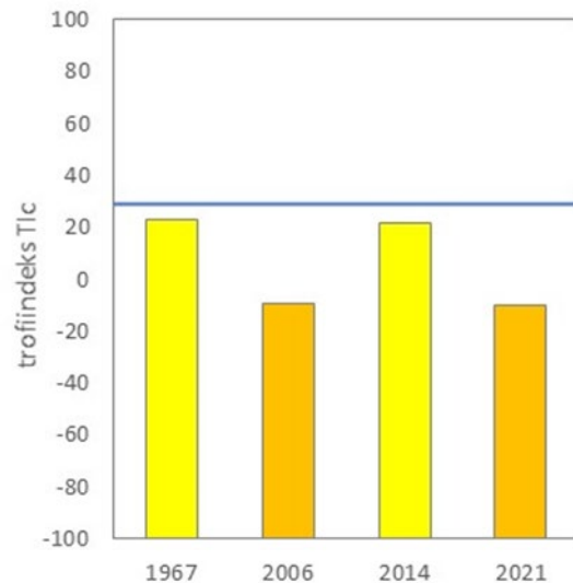
Figur 9. Endring i Tic-indeksen i perioden 1967-2021. Grense mellom god og moderat tilstand er markert.
