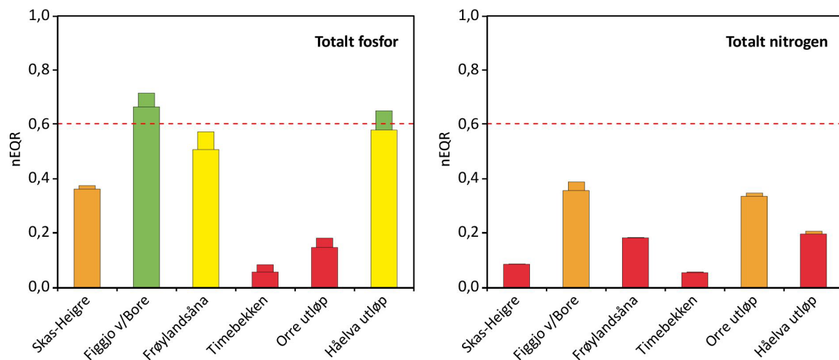
Figur 15. Tilstand i elver i 2021, basert på fosfor- og nitrogeninnhold (beregnete nEQR-verdier). Søyler for medianverdier vises bak søyler for gjennomsnittsverdier.
