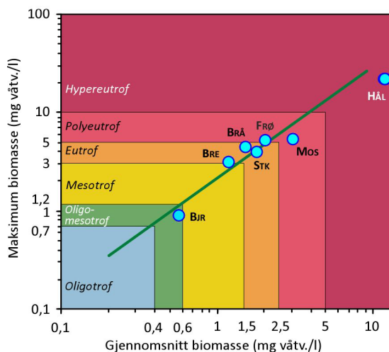
Figur 1. Plantep plankton og trofegrad i 2021. Regresjonslinje fra Brettum & Andersen (2005).
