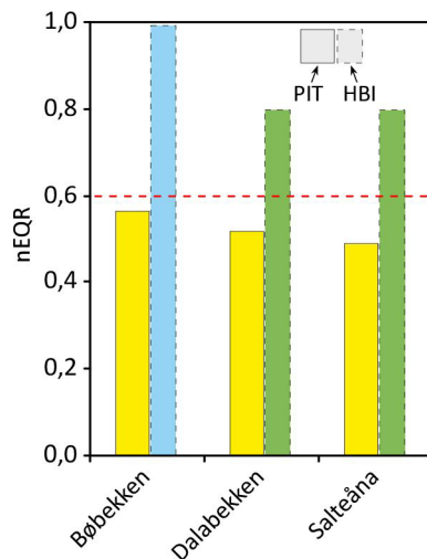
Figur 11. Tilstand basert på begroing i undersøkte elver i 2021 (nEQR for påvekstalger [PIT] og heterotrof begroing [HBI]). [Påvekstalger vist i søyler til venstre med heltrukken kantlinje, og heterotrof begroing i søyler til høyre med stiplede kantlinje.]
