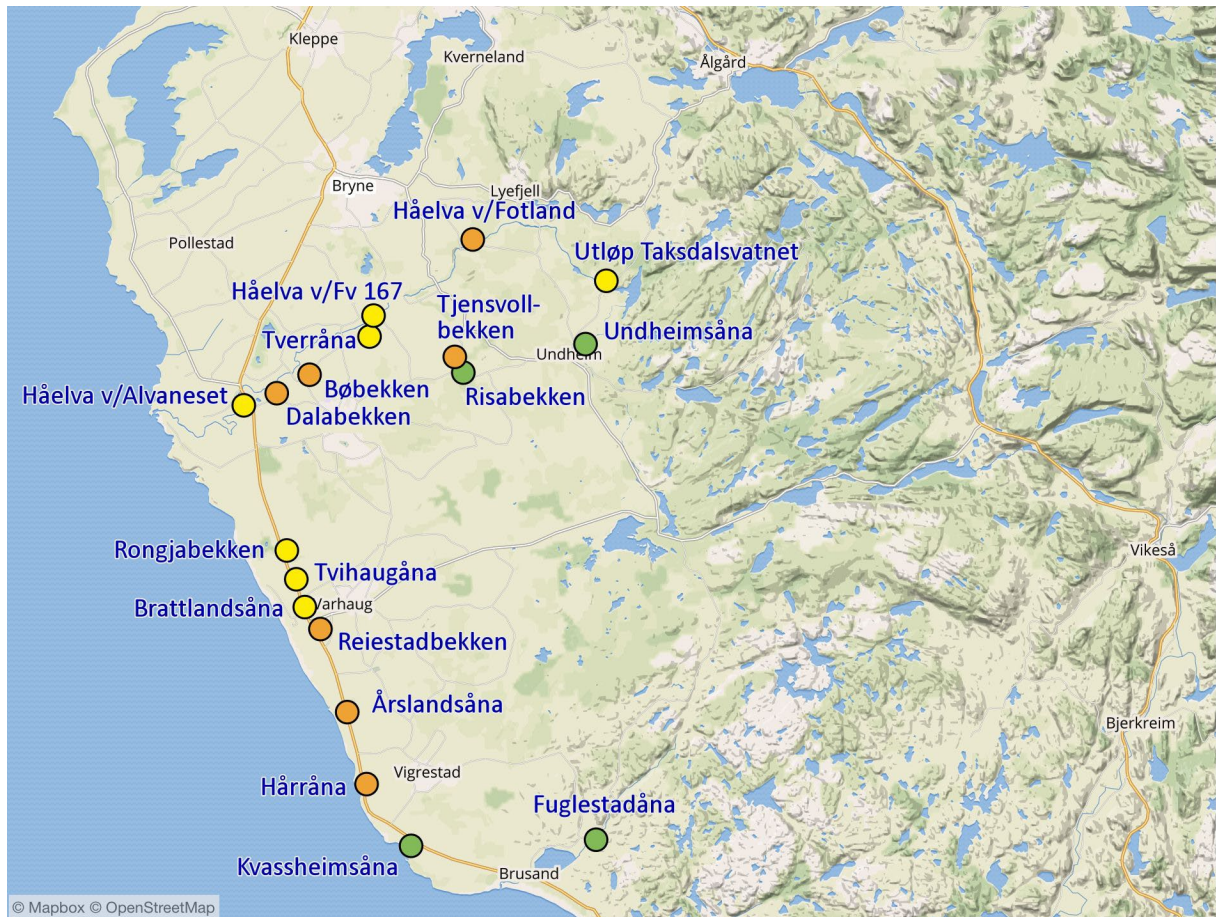
Figur 12. Elvelokaliteter hvor bunndyr ble undersøkt i 2021. (Økologisk tilstand angitt med fargekode.)
