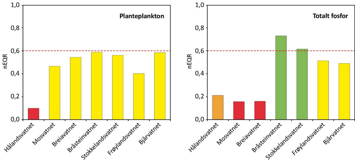
Figur 3. Planteplankton og totalt fosfor i innsjøene i 2020 (beregnete nEQR-verdier).
