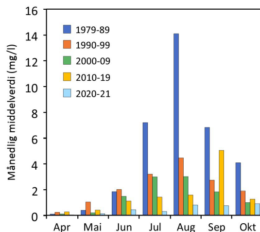
Figur 23. Biomasse av blågrønnalger i Frøylandsvatnet.
