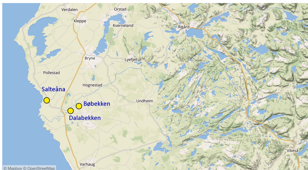
Figur 10. Elvelokaliteter hvor begroing ble undersøkt i 2021. (Økologisk tilstand er angitt med fargekode.)
