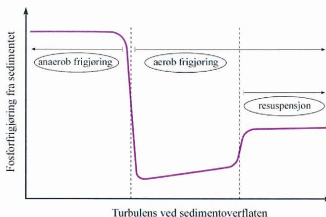
Figur 11. Effekter av turbulens på fosforfrigjøring fra sedimentet (omarbeidet etter Scheffer 1998).
