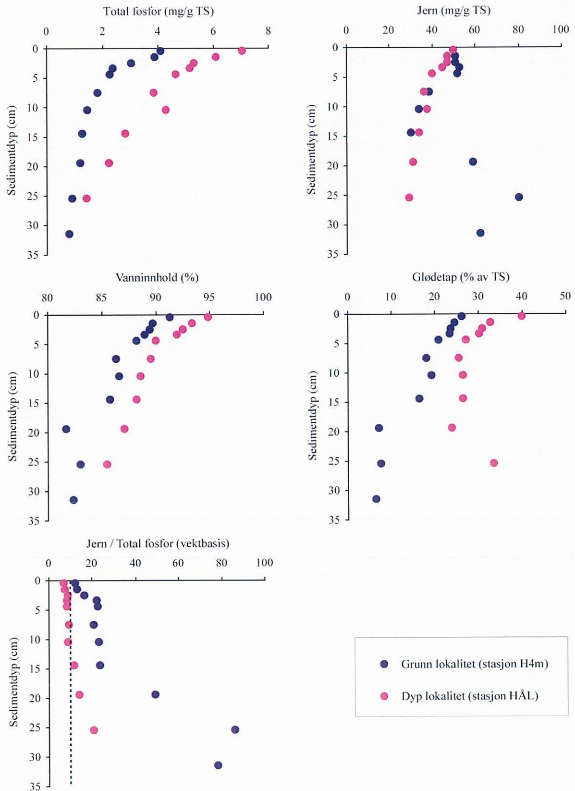
Figur 7. Fosfor, jern, vanninnhold, glødetap og forhold mellom jern og fosfor i grunntvannssediment og dypvannssediment i Hålandsvatnet.
