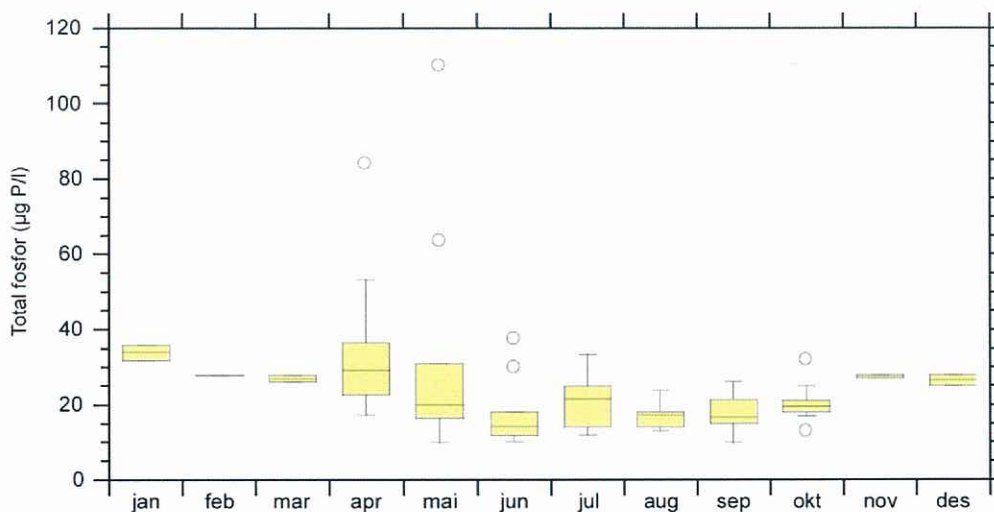
Figur 12. Box-plot som viser sesongutvikling for total fosfor i overflatevann i Hålandsvatnet.
