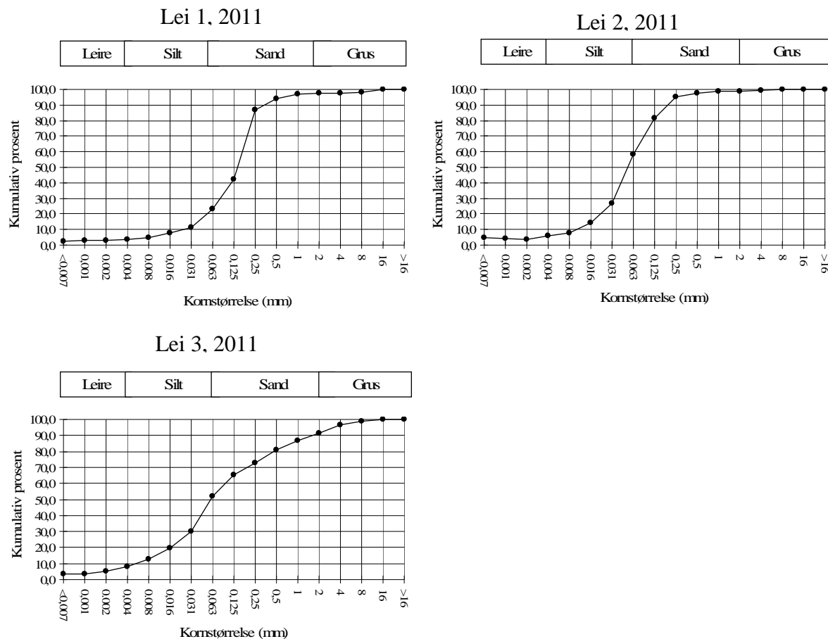
Figur 3.1. Kornfordeling (mm) langs x-aksen og kumulativ vektprosent langs y-aksen av sedimentprøver fra stasjonene Lei 1, Lei 2 og Lei 3.
