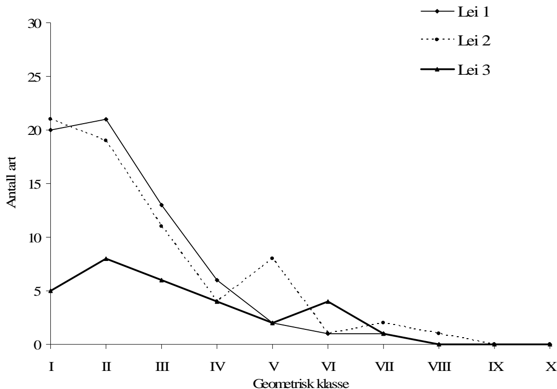
Figur 3.4. Antall arter langs (y-akse) er plottet mot geometriske klasser (x-akse) i prøvene.
