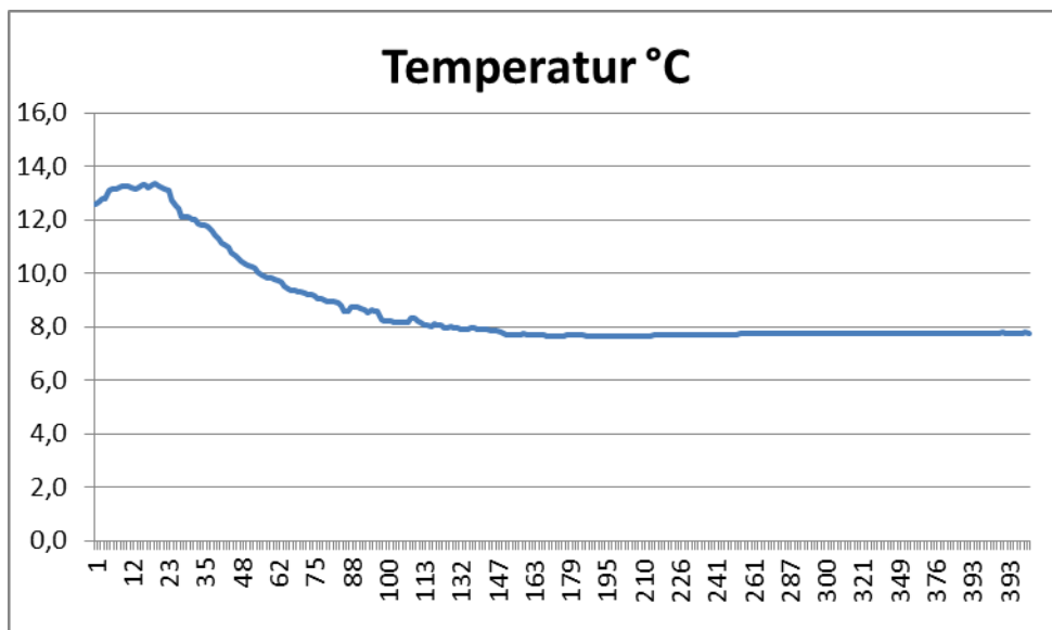
Figur 3.1 Temperatur fra overflate til bunn.
