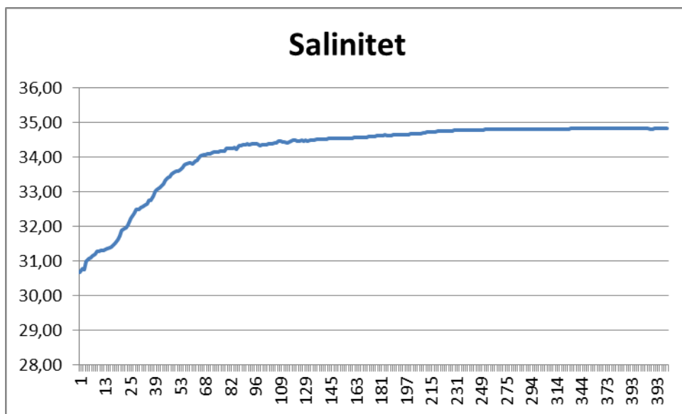
Figur 3.2 Salinitet (i promille) fra overflate til bunn.
