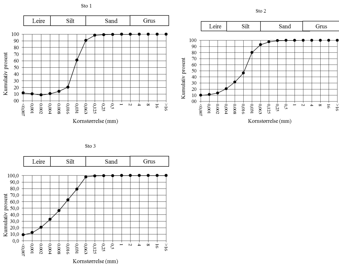
Figur 3.3. Kornfordeling (mm) langs x-aksen og kumulativ vektprosent langs y-aksen av sedimentprøver fra stasjonene Sto 1, Sto 2 og Sto 3.
