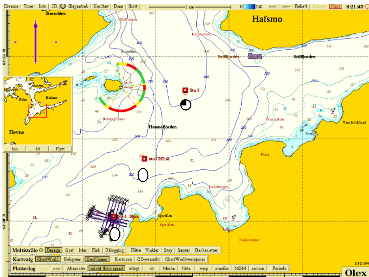
Figur 2.1. Oversiktskart (innfelt bilde) og mer detaljert kart ved lokaliteten Stokkvika. Vurdering av miljøforholdene er vist som kakediagram, der ○ = svært bra, ◐ = bra, ◑ = middels, ◒ = dårlige miljøforhold og ◓ = dødt. Kartkilde: Olex
