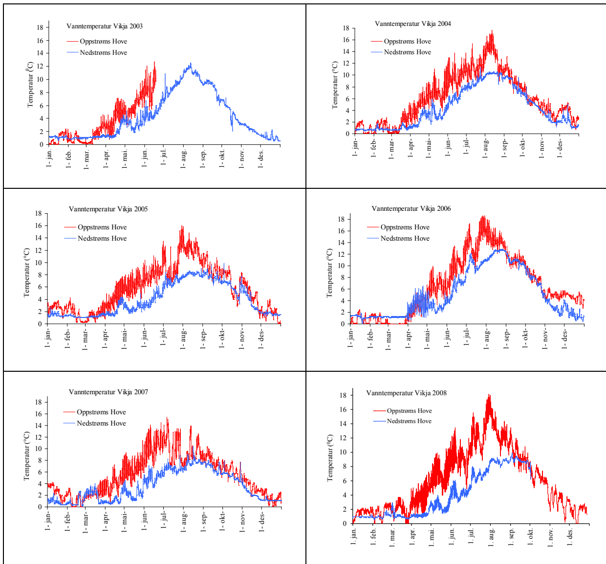
Figur 16. Vanntemperatur registrert annenhver time i Vikja oppstrøms og nedstrøms Hove kraftstasjon i perioden 2003-2008. I 2003 finnes det kun data t.o.m. 17. juni oppstrøms Hove.
