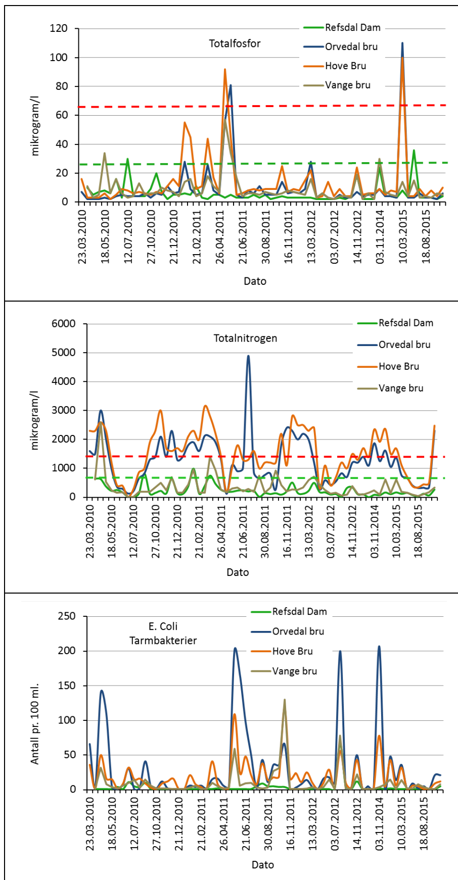
Figur 24. Konsentrasjoner av totalfosfor, totalnitrogen og E. coli (tarmbakterier) i Vikja prøvetatt ved Refsdal dam, Orvedal bru, Hove bru og Vange bru i perioden 2010-2015. Rød stiplede linje angir en svært dårlig miljøtilstand, mens grønn linje angir en god miljøtilstand.
