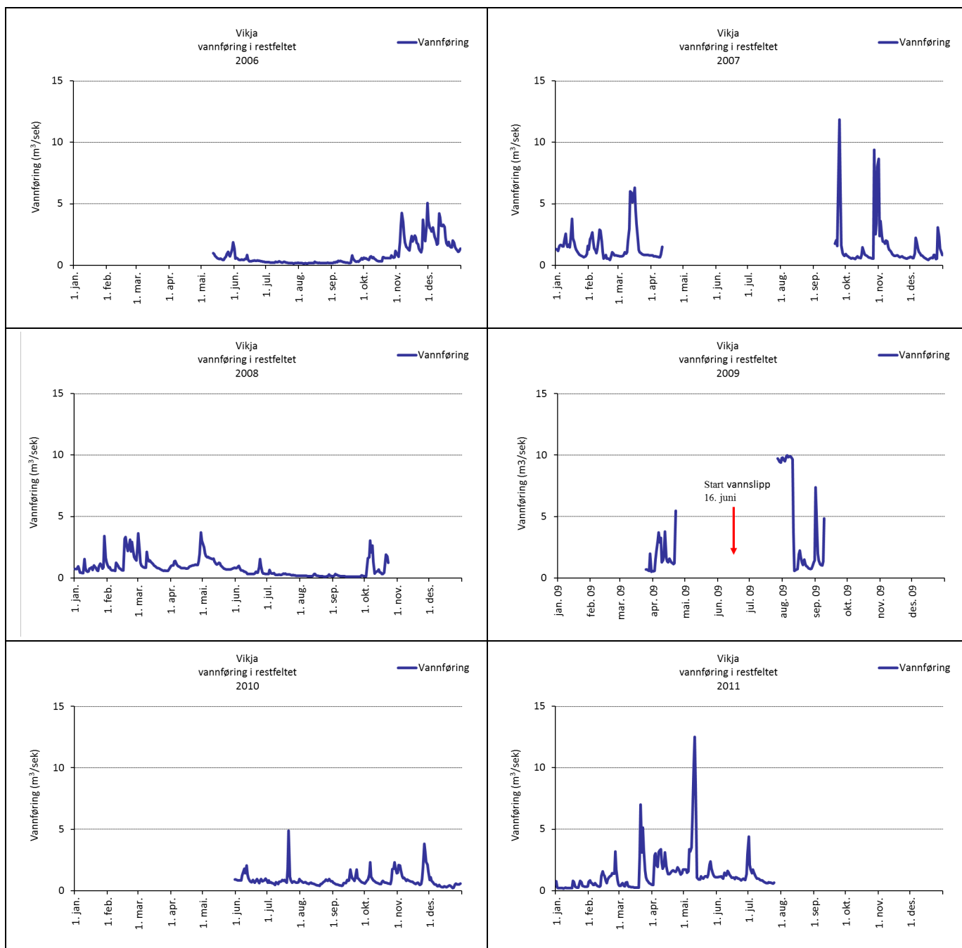
Figur 22. Vannføring i restfeltet i Vikja målt rett oppstrøms utløpet av Hove kraft. Fra og med 16. juni 2009 ble det startet slipp av vann, maksimum 200 l/s.
