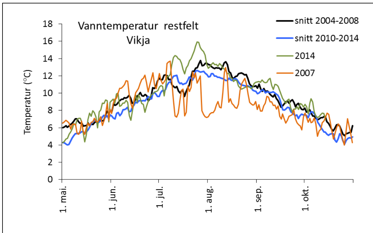
Figur 17. Døgnmiddel for perioden 2004-2005 (svart linje) og tilsvarende for 2010-2014 (blå linje) i restfeltet i Vikja. I tillegg er døgntemperaturene for 2014 (grønn linje) og 2007 (oransje linje) vist. Slipp av vann fra dammen ved Refsdal i restfeltet startet i 2009.
