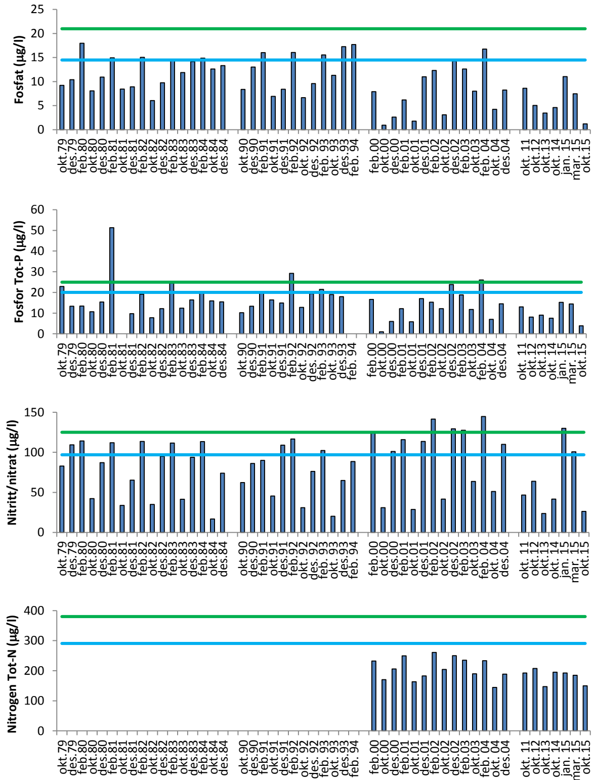
Figur 3.1.7 Gjennomsnittlig konsentrasjon av fosfat, nitrat/nitritt, total fosfor og total mengde nitrogen i prøver fra overflatelaget (0-10 m dyp) ved St. 121 i vinterhalvåret tatt i perioden 2015 med historiske data. Miljødirektoratet grense for tilstandsklasser I og II for vinterhalvåret er markert med henholdsvis blå og grønn linje.
