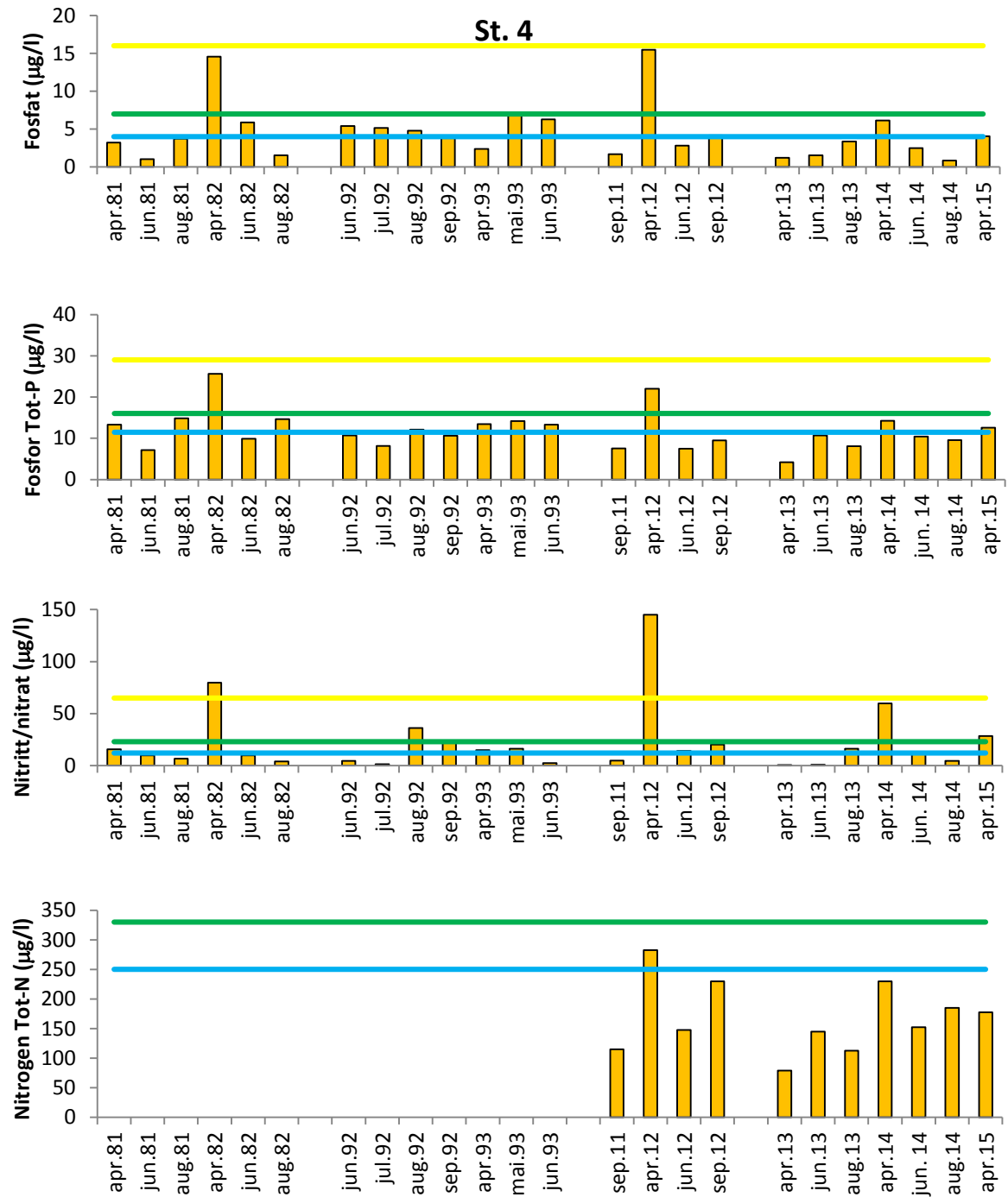
Figur 3.4.4 Gjennomsnittlig konsentrasjon av fosfat, nitrat/nitritt, total fosfor og total mengde nitrogen i prøver fra overflatelaget (0-10 m dyp) ved St. 4 i sommerhalvåret fra 2015 med historiske data. Miljødirektoratets grense for tilstandsklasser I, II og III for sommerhalvåret er markert med henholdsvis blå, grønn og gul linje.
