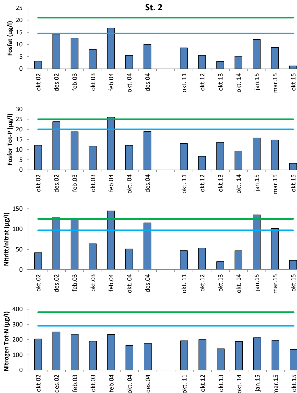
Figur 3.1.3 Gjennomsnittlig konsentrasjon av fosfat, nitrat/nitritt, total fosfor og total mengde nitrogen i prøver fra overflatelaget (0-10 m dyp) ved St. 2 i vinterhalvåret tatt i perioden 2015 med historiske data. Miljødirektoratet grense for tilstandsklasser I og II for vinterhalvåret er markert med henholdsvis blå og grønn linje.
