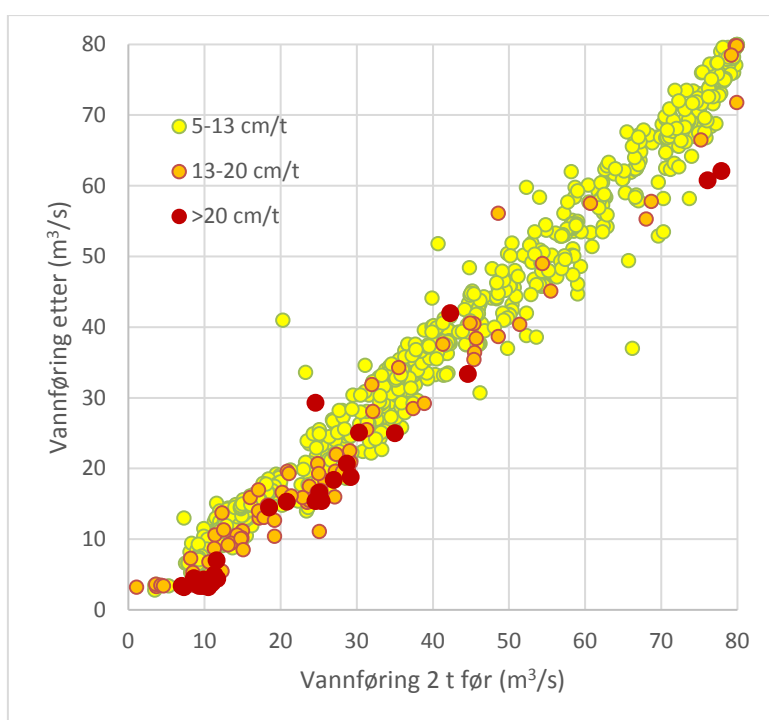
Figur 13. Driftsvannføring i Årøy kraftverk før og etter hurtige vannstandsendinger i Årøyelva i perioden 2013 og frem til 21. mai 2017.
