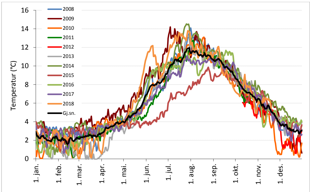
Figur 30. Gjennomsnittlig vanntemperatur per døgn i Øyreselva i 2008-2018.
