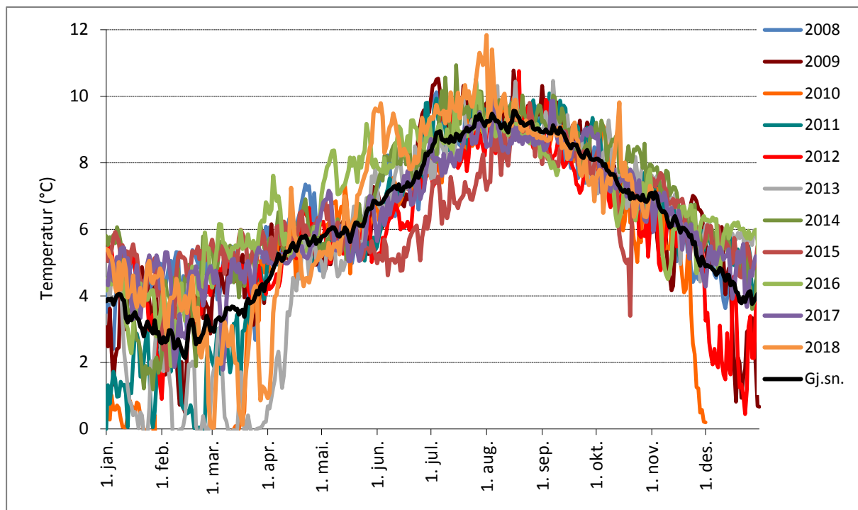
Figur 9. Døgnmiddeltemperaturer fra loggere i Sima i perioden 2008-2018. Temperaturer under 0 grader tyder på at loggeren ved flere anledninger har vært tørrlagt i perioder på vinteren.
