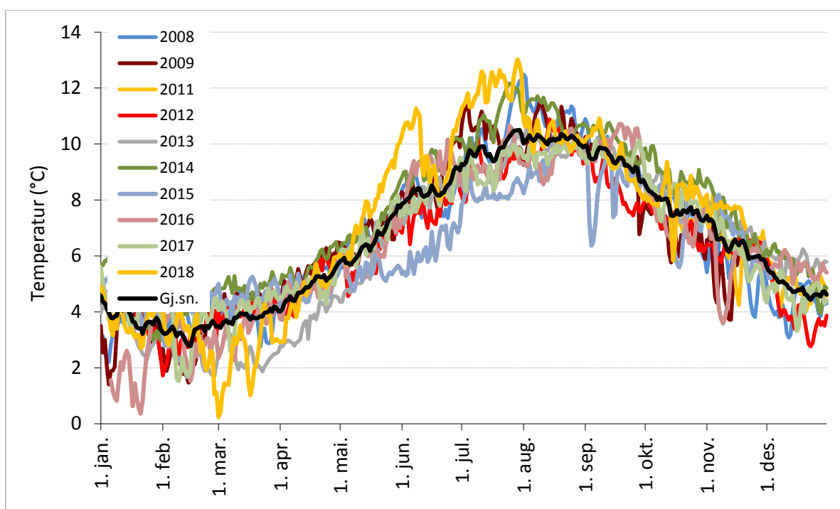
Figur 36. Gjennomsnittlig vanntemperatur per døgn i Austrepollelva for deler av perioden 2008-2018.
