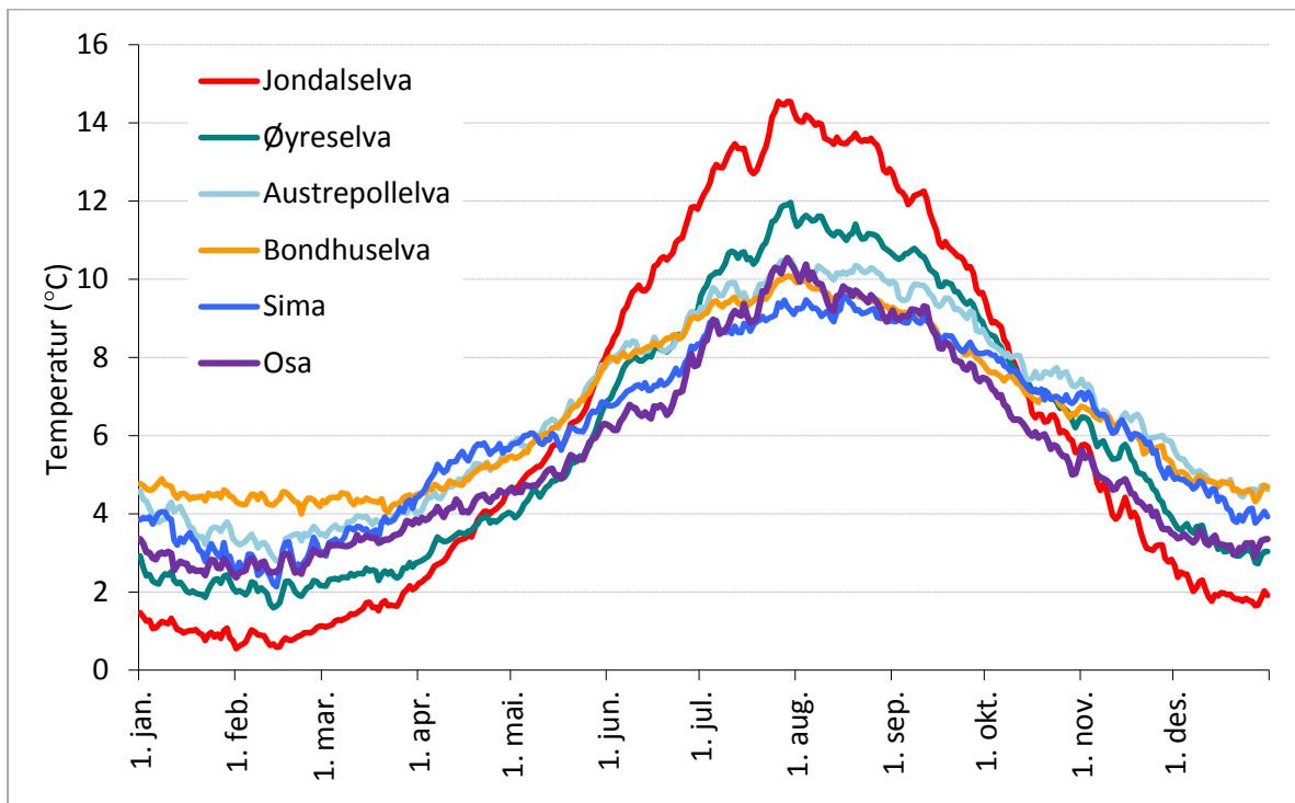
Figur 3. Gjennomsnittlig vanntemperatur på døgnnivå fra de seks regulerte elvene i Hardanger i perioden 2007-2018.
