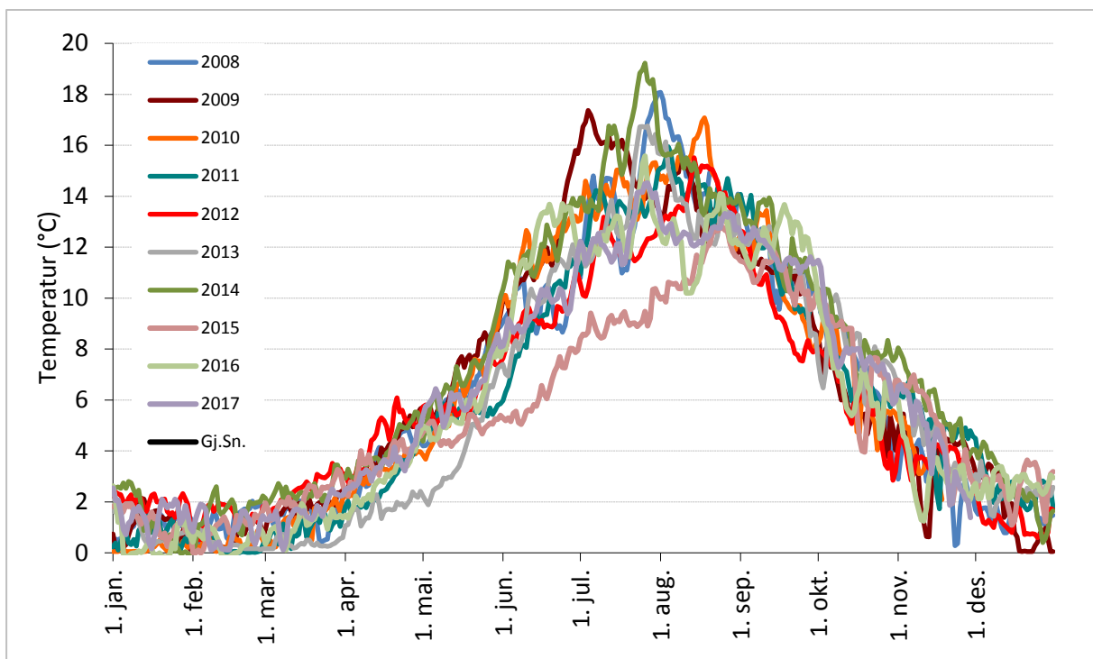
Figur 24. Døgnmiddeltemperatur i Jondalselva i perioden 2008-2017.
