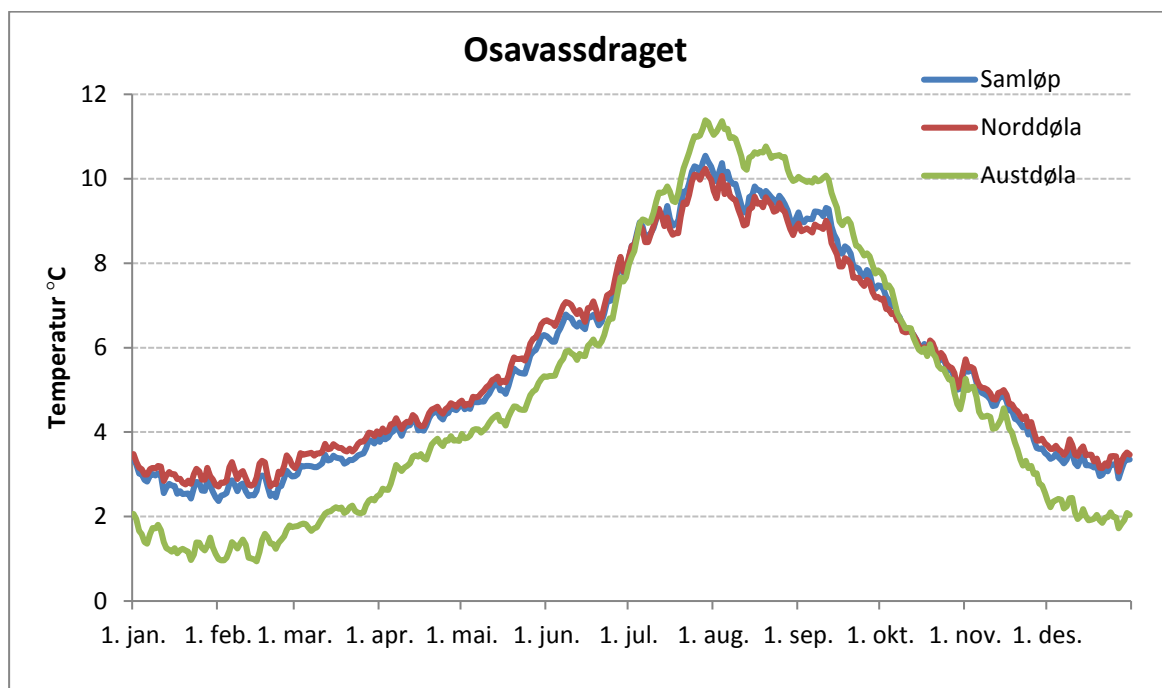
Figur 15. Døgnmiddeltemperaturer (gjennomsnitt for døgn) i de ulike vassdragsavsnittene i Osavassdraget i perioden 2008-2018.
