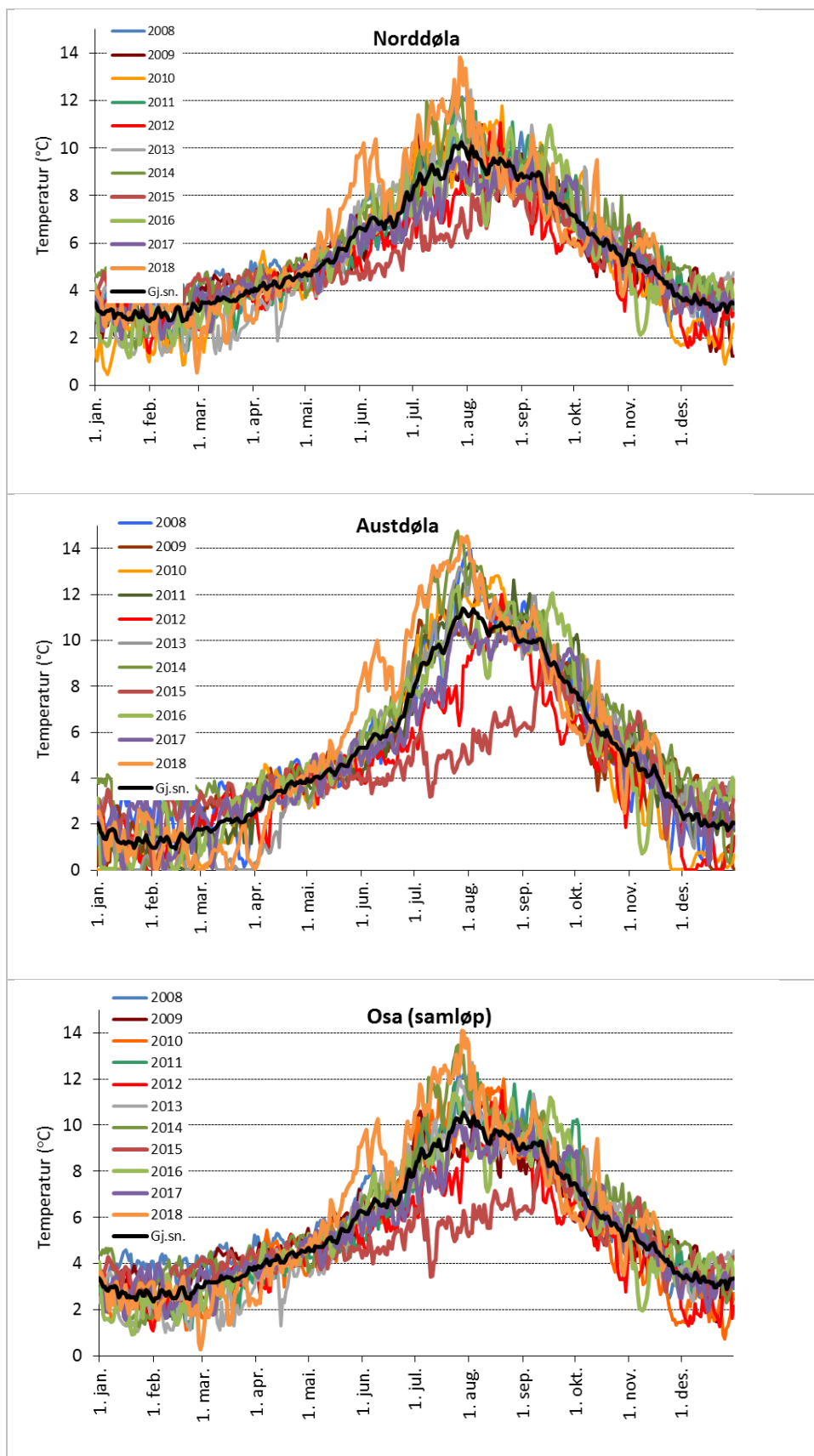
Figur 16. Døgnmiddeltemperatur i Norddøla (øverst), Austdøla (midten) og samløpet (nederst) i 2008-2018.
